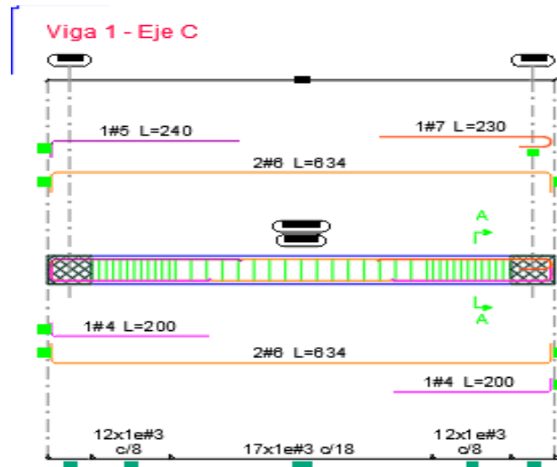
Ilustración 6. Disposición de refuerzo viga C (3-4)
