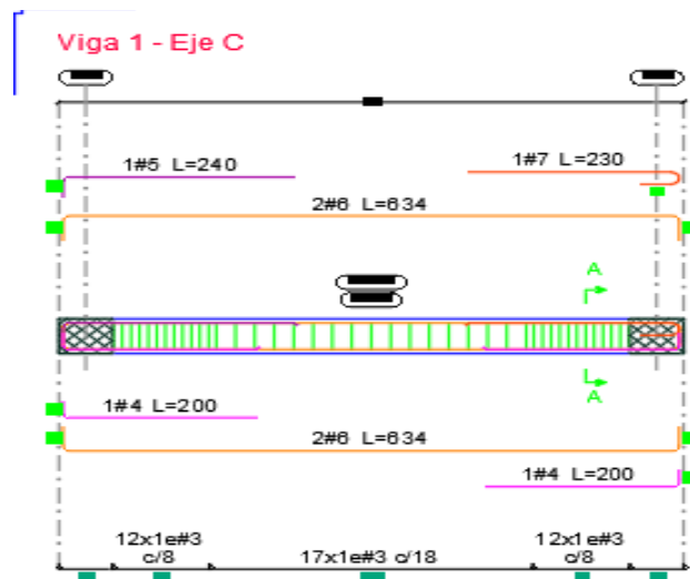
Ilustración 16. Disposición de refuerzo viga 4 (D-D').
