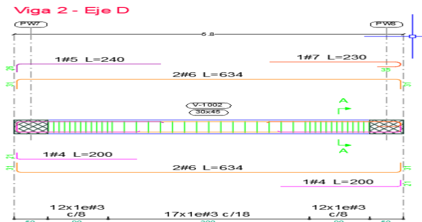
Ilustración 7. Disposición de refuerzo viga D (3-4)
