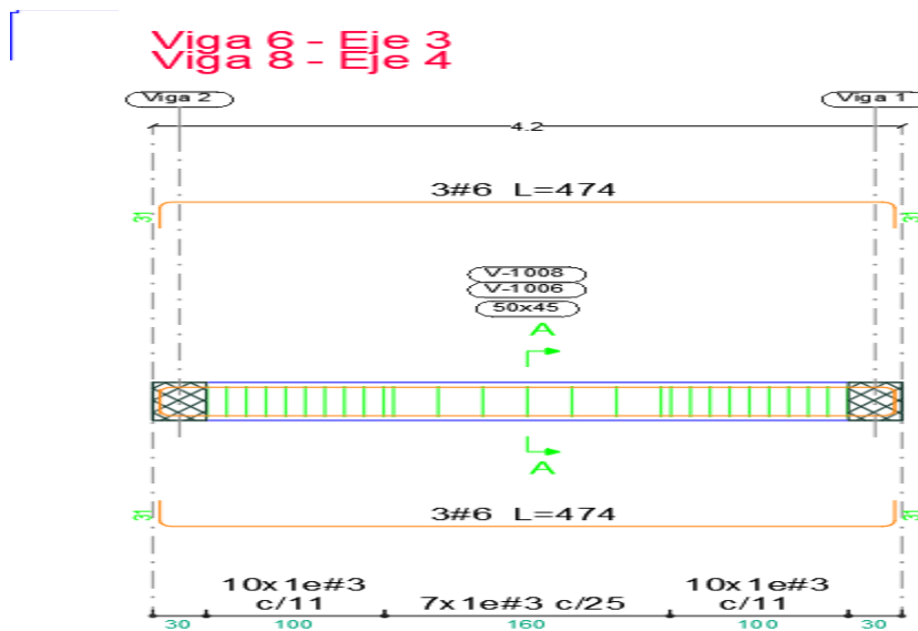
Ilustración 15. Disposición de refuerzo viga 4 (C-D)
