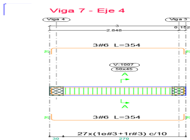
Ilustración 17. Disposición de refuerzo viga 4 (D'-E)
