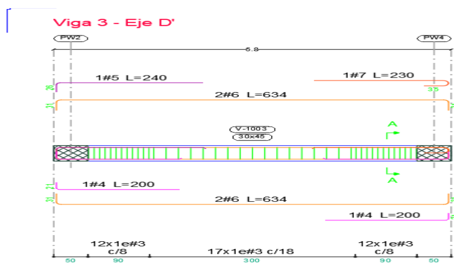
Ilustración 9. Disposición de refuerzo viga D´(3-4)
