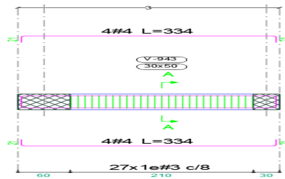
Ilustración 14. Disposición de refuerzo viga 3' (D' - E)
