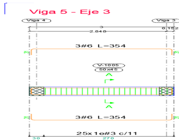
Ilustración 13. Disposición de refuerzo viga 3 (D'-E)
