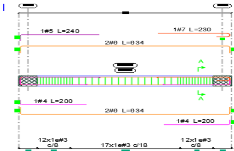
Ilustración 8. Disposición de refuerzo viga D”(3-4)
