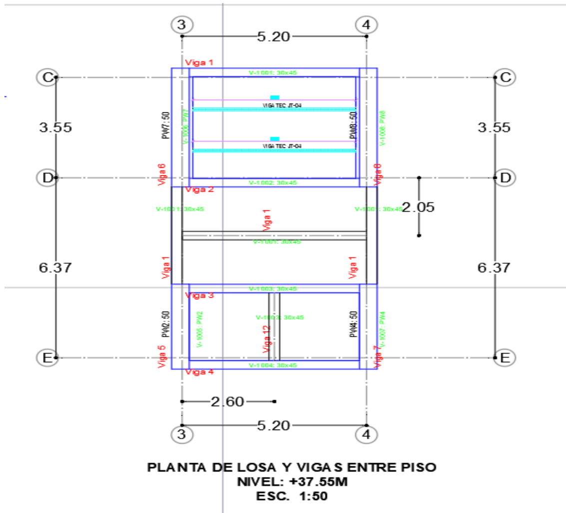
Ilustración 3. Disposición de vigas joist entre piso 10 N+37.55
