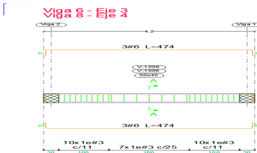
Ilustración 11. Disposición de refuerzo viga 3(C-D)
