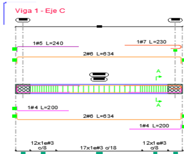
Ilustración 12. Disposición de refuerzo viga 3' (D-D')
