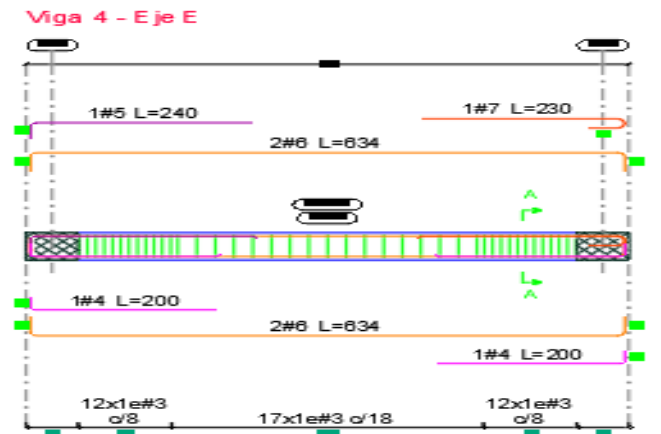
Ilustración 10. Disposición de refuerzo viga E (1-6)
