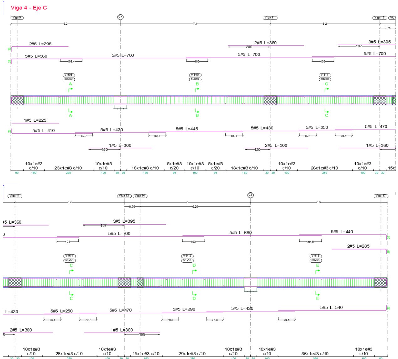
Ilustración 14. Disposición de refuerzo viga C
