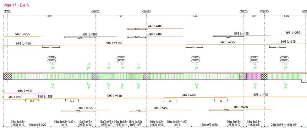
Ilustración 26. Disposición de refuerzo viga 6 (A-E)
