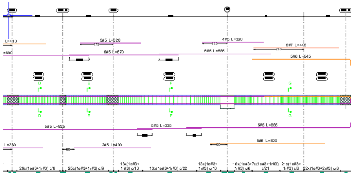
Ilustración 17. Disposición de refuerzo viga E (1-6)
