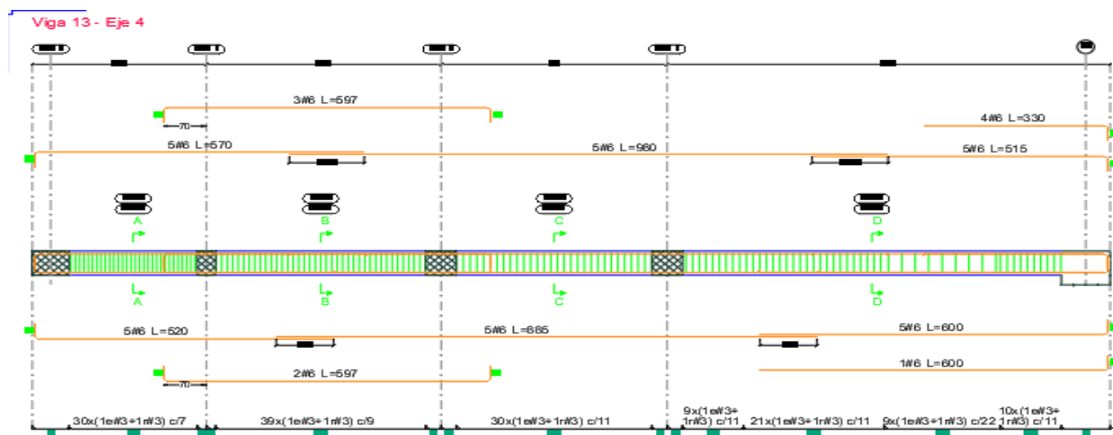
Ilustración 22. Disposición de refuerzo viga 4 (B-E)
