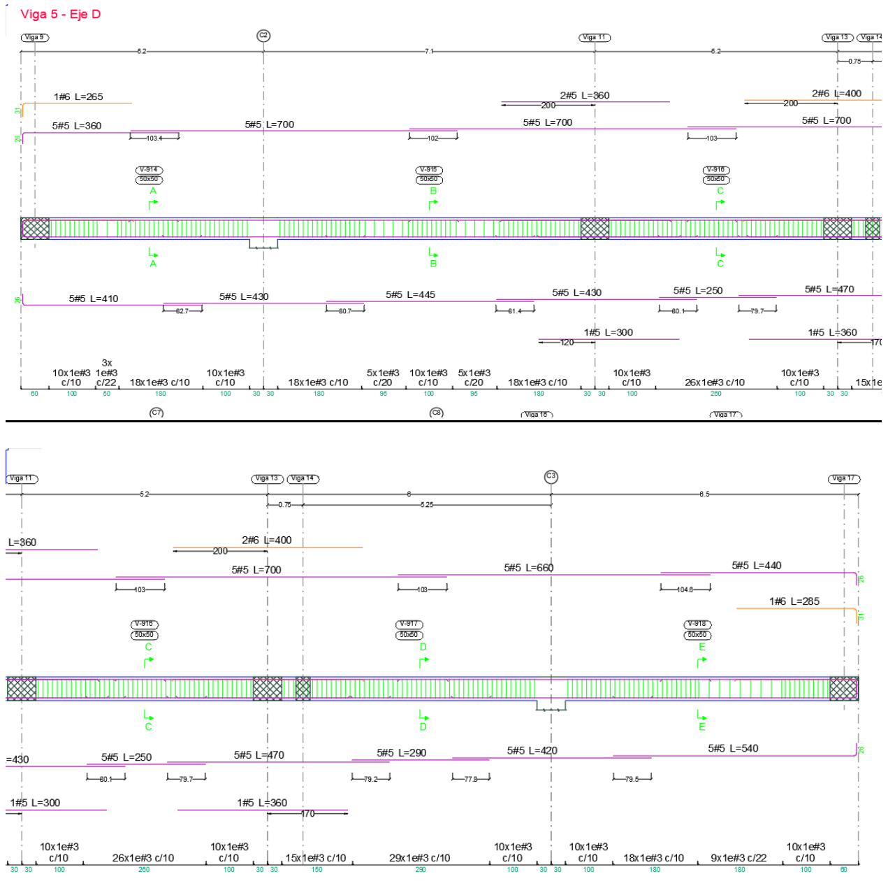
Ilustración 15. Disposición de refuerzo viga D (1-6)
