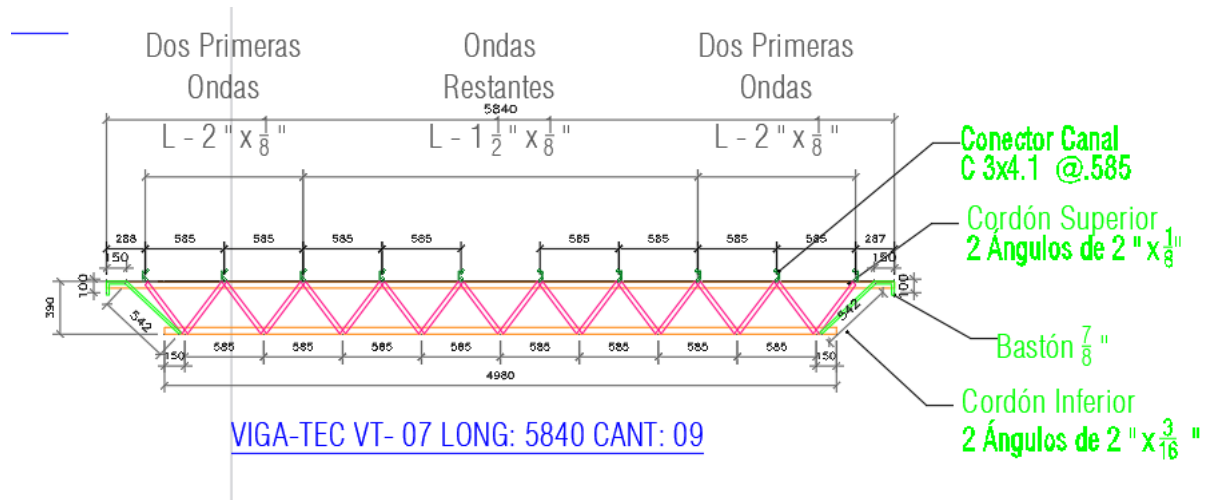
Ilustración 9. Detalle joist VT 07.
