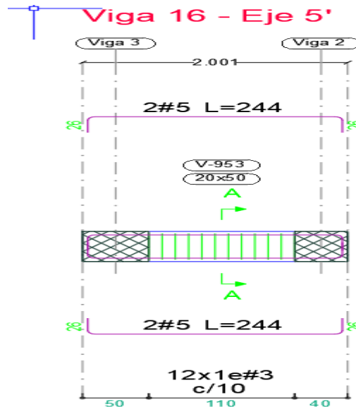
Ilustración 25. Disposición de refuerzo viga 5' (B-E)
