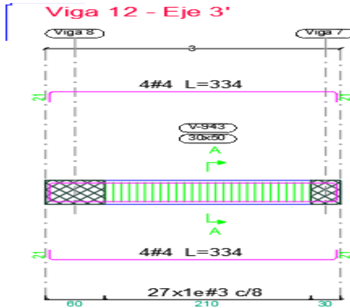
Ilustración 21. Disposición de refuerzo viga 3*(B-E)
