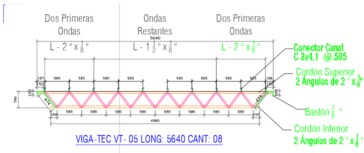
DETALLE VIGA TEC VT 05
