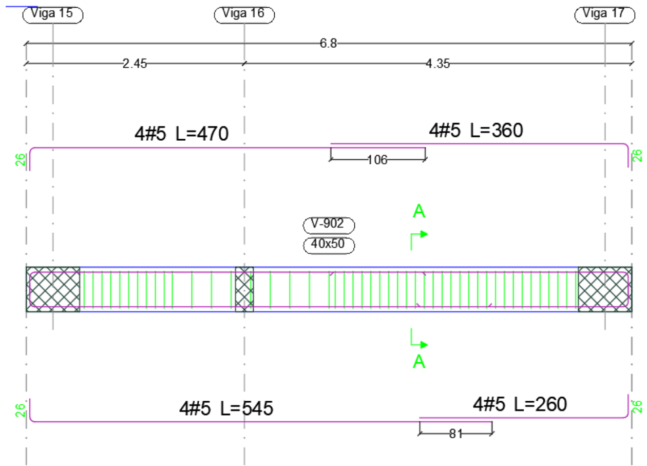
Ilustración 12. Disposición de refuerzo viga A'
