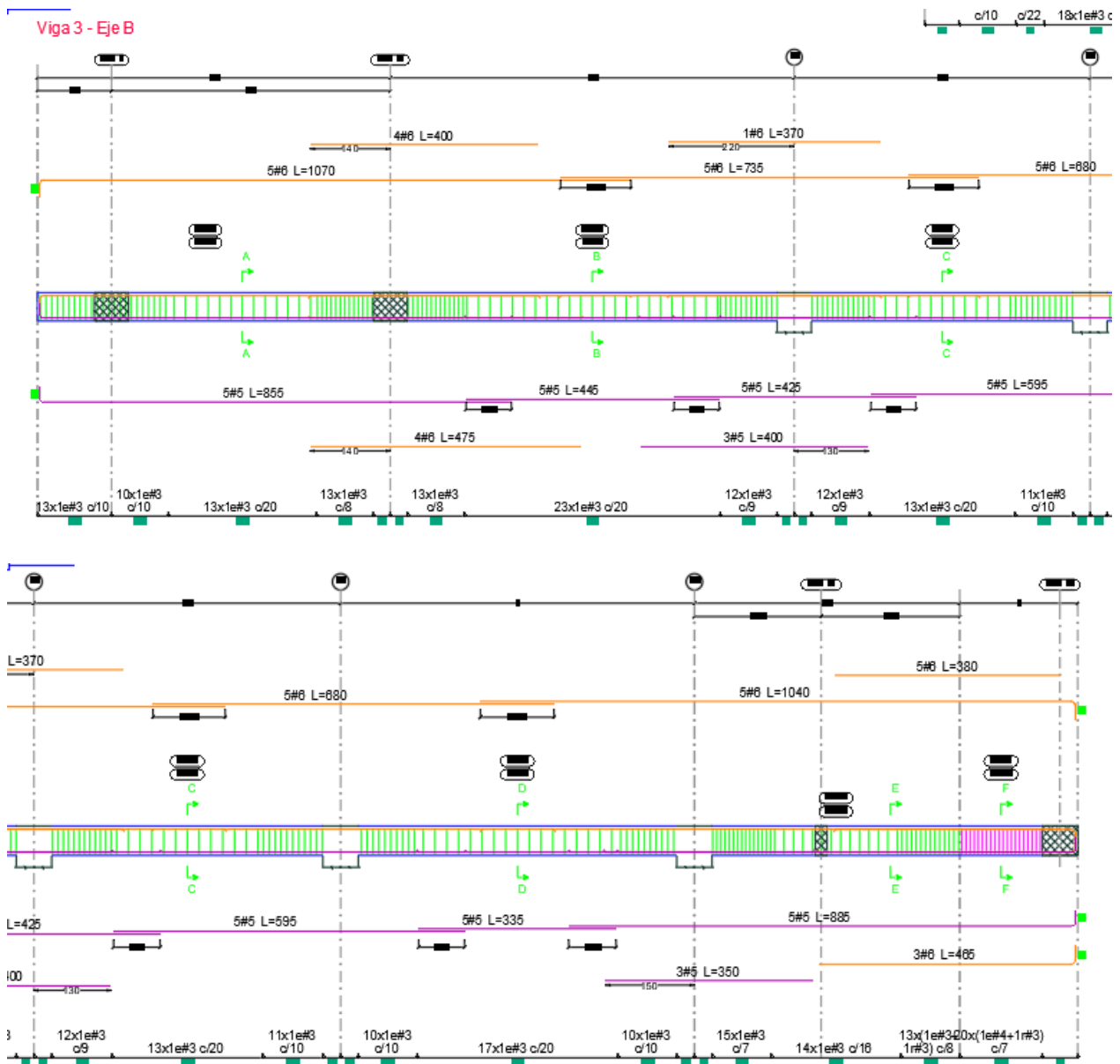
Ilustración 13. Disposición de refuerzo viga B
