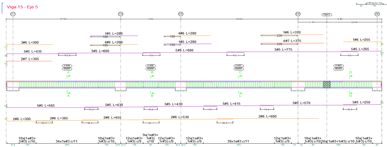
Ilustración 24. Disposición de refuerzo viga 5 (B-E)
