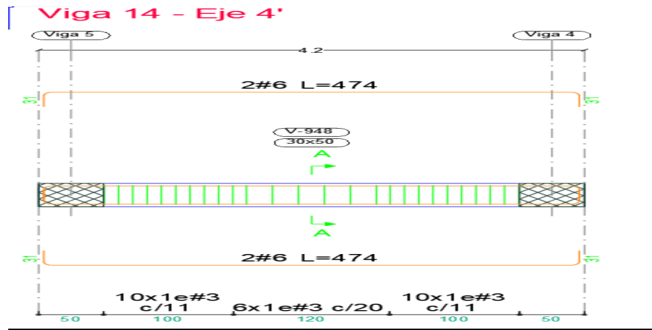
Ilustración 23. Disposición de refuerzo viga 4 (C-D)
