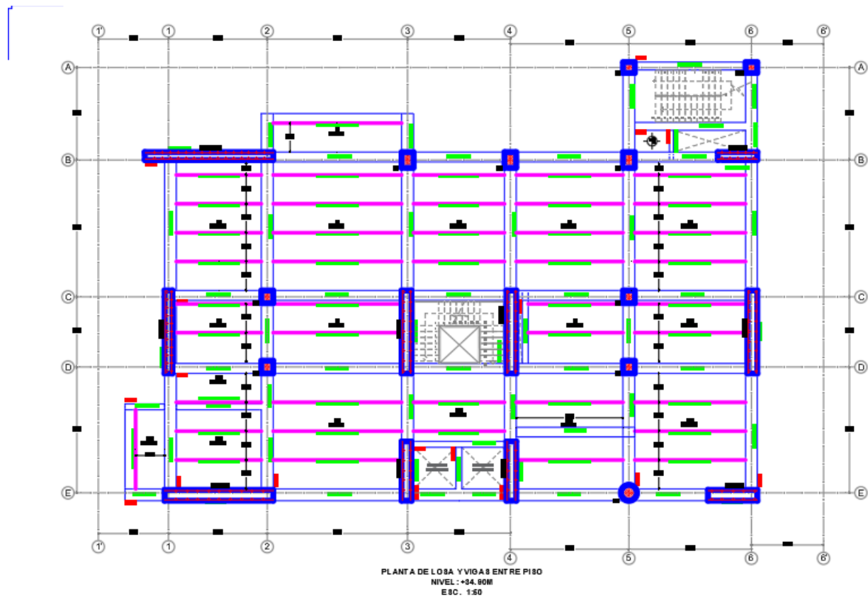
Ilustración 10. Detalle vigas de entrepiso 9 N+34.90
