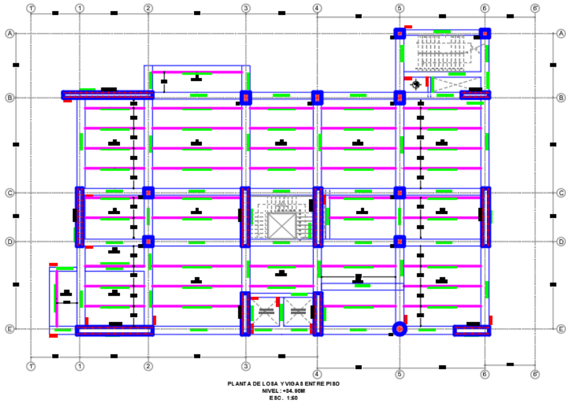
Ilustración 3. Disposición de vigas joist entre piso 9 N+34.90
