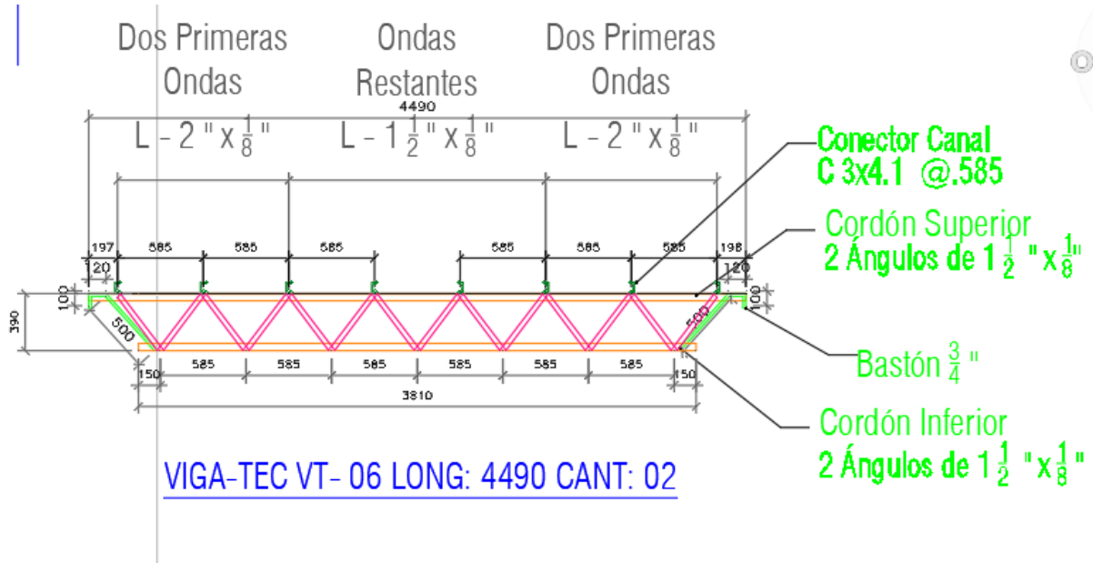
Ilustración 8. Detalle joist VT 06.
