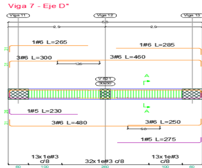
Ilustración 31. Disposición de refuerzo viga D' (3-4)
