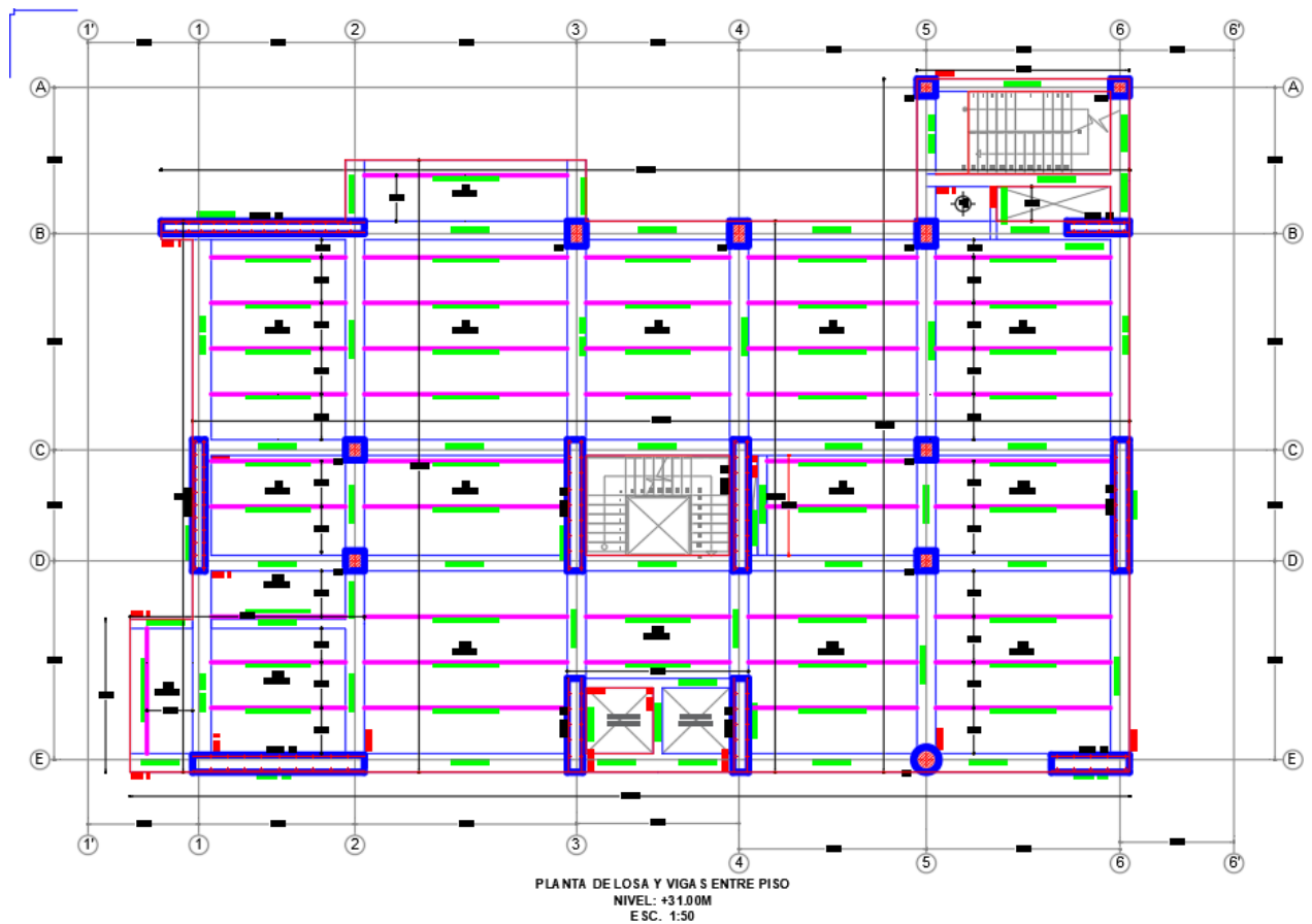
Ilustración 24. Detalle vigas de entrepiso 8 N+31,00
