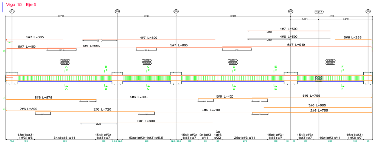
Ilustración 39. Disposición de refuerzo viga 5 (B-E)
