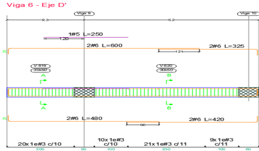
Ilustración 30. Disposición de refuerzo viga D' (1'-2)
