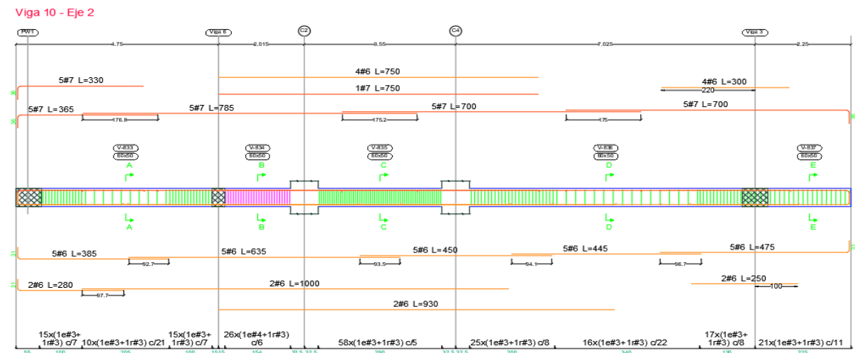
Ilustración 34. Disposición de refuerzo viga 2 (B-E)
