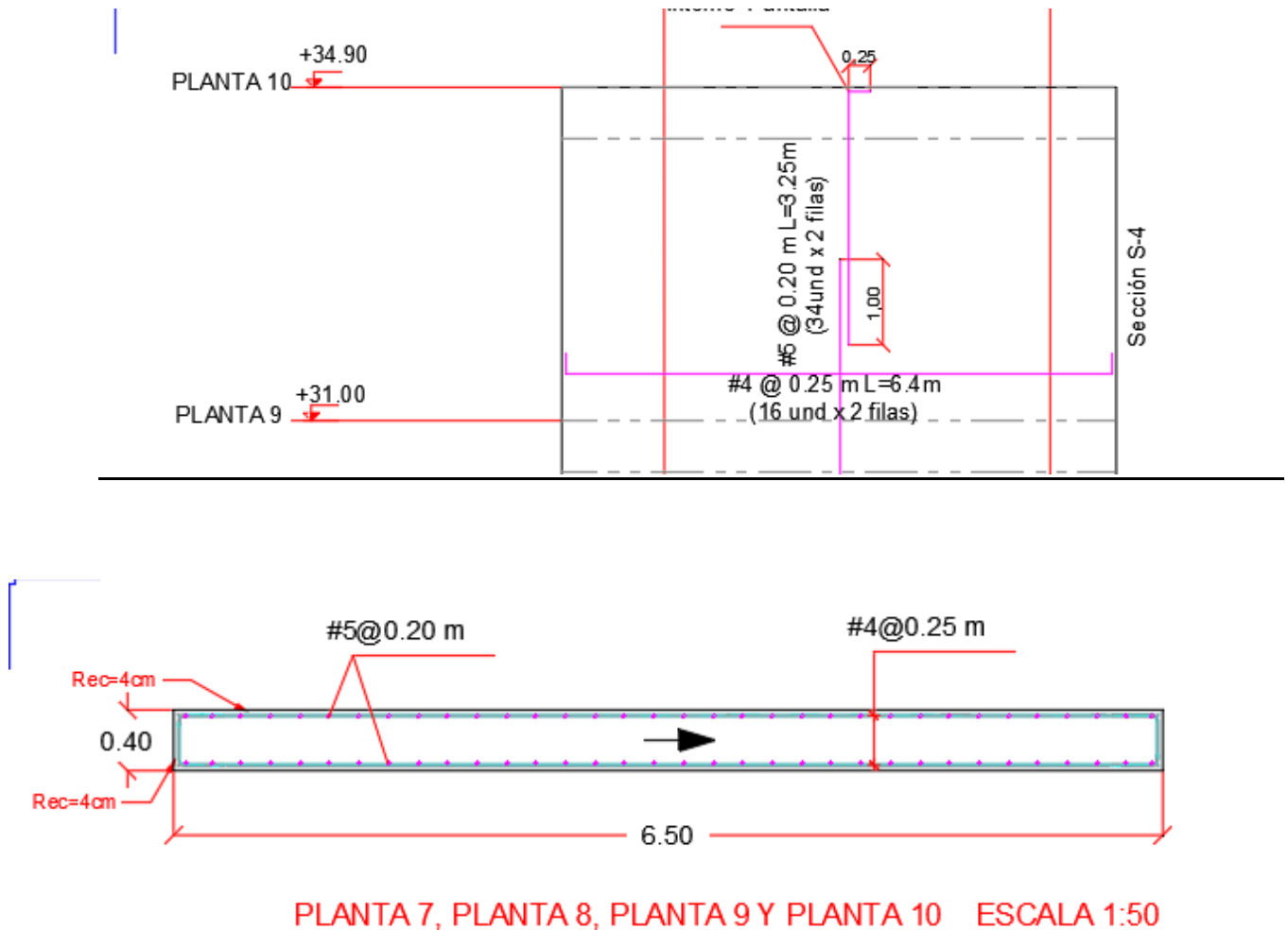
Ilustración 16. Disposición acero de refuerzo pantalla PW10.
