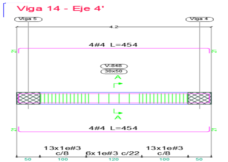
Ilustración 38. Disposición de refuerzo viga 4 (C-D)
