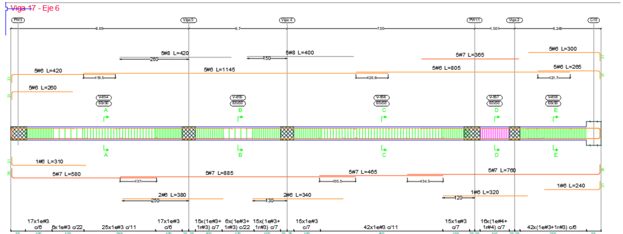
Ilustración 41. Disposición de refuerzo viga 6 (A-E)
