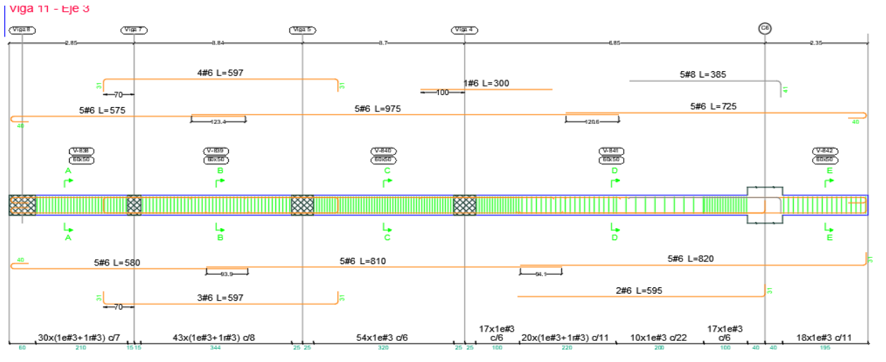
Ilustración 35. Disposición de refuerzo viga 3(B-E)
