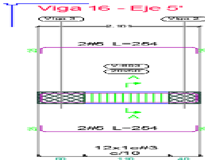
Ilustración 40. Disposición de refuerzo viga 5' (B-E)
