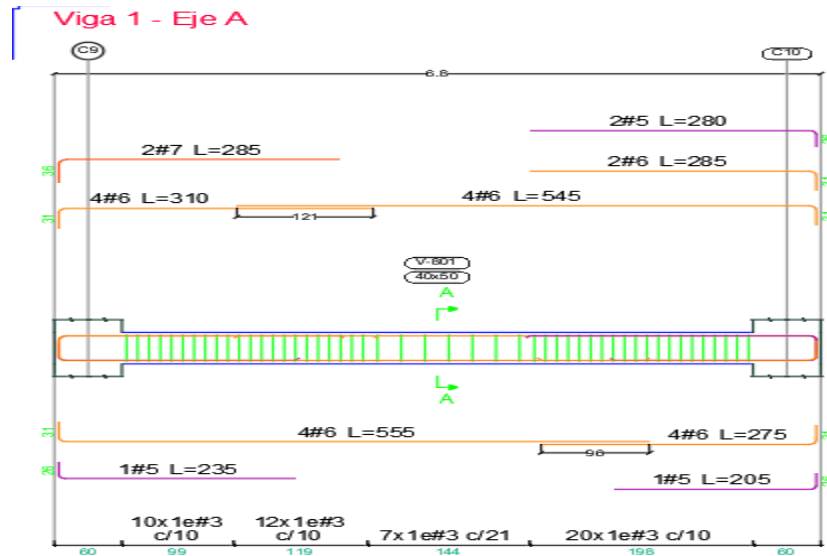
Ilustración 25. Disposición de refuerzo viga A.
