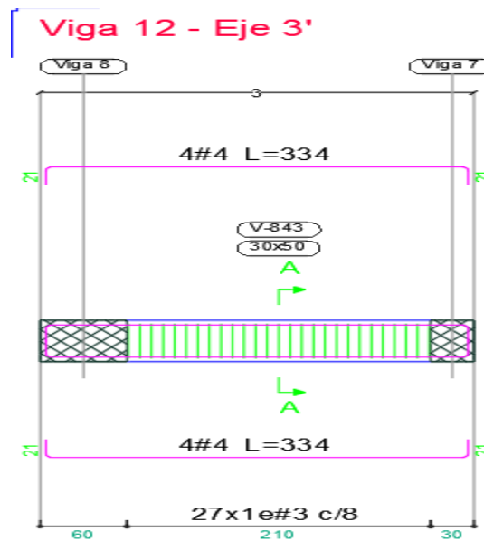
Ilustración 36. Disposición de refuerzo viga 3*(B-E)
