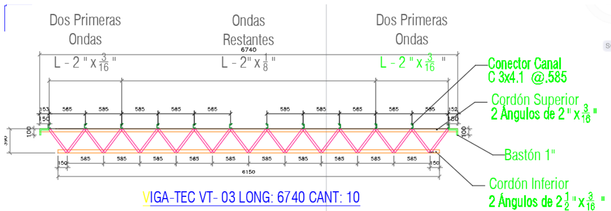
Ilustración 19. Detalle joist VT 03.
