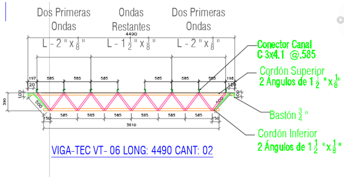
Ilustración 22. Detalle joist VT 06.
