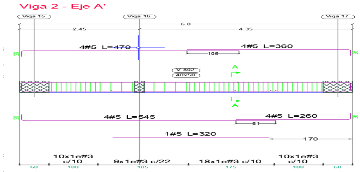
Ilustración 26. Disposición de refuerzo viga A'
