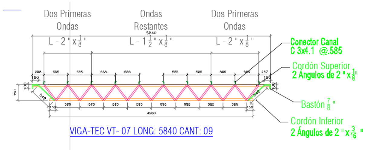
Ilustración 23. Detalle joist VT 07.
