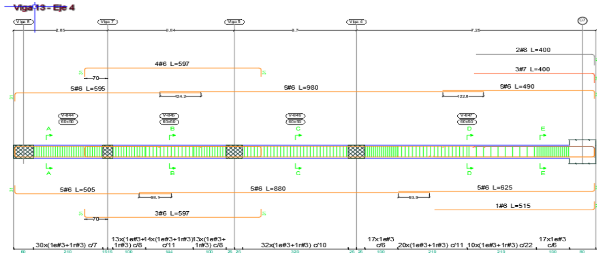
Ilustración 37. Disposición de refuerzo viga 4 (B-E)
