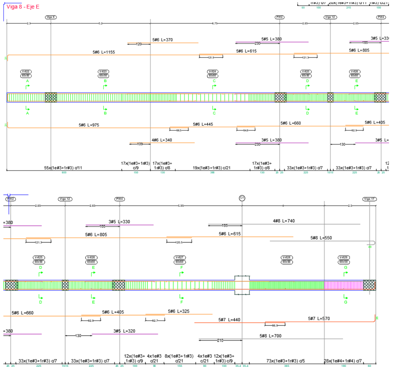
Ilustración 32. Disposición de refuerzo viga E (1-6)
