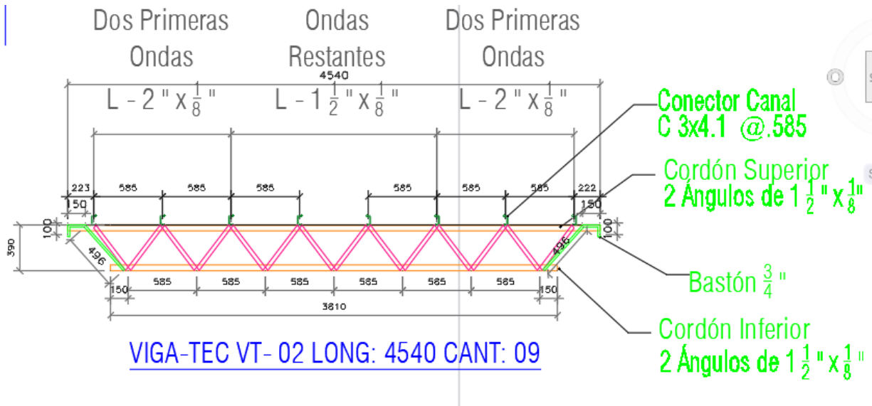
Ilustración 18. Detalle joist VT 02
