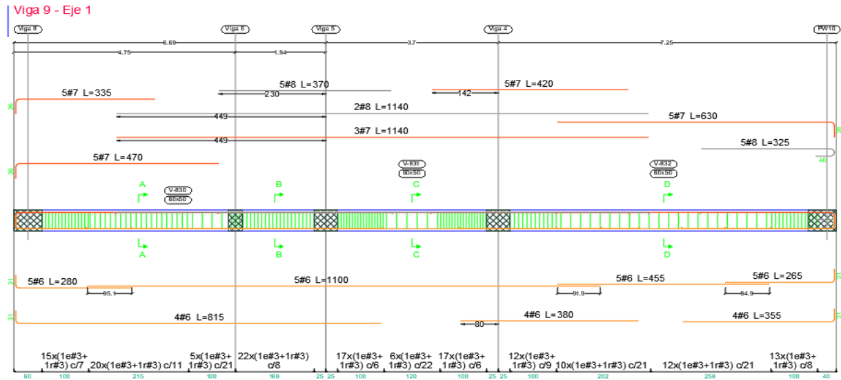
Ilustración 33. Disposición de refuerzo viga 1 (B-E)
