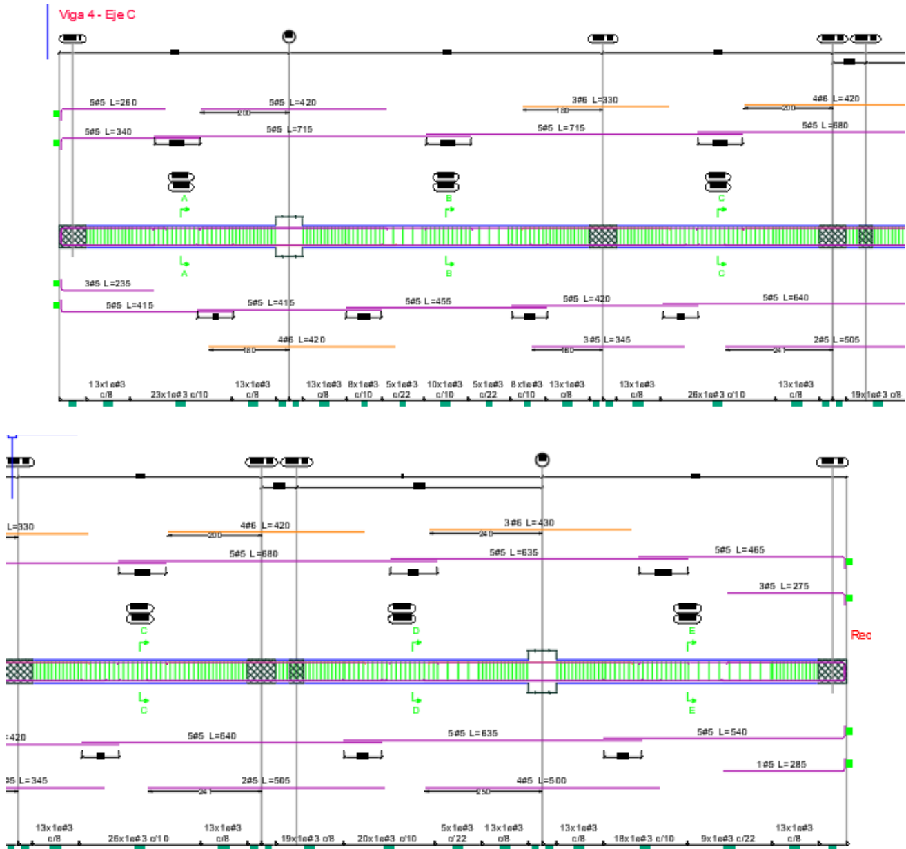
Ilustración 28. Disposición de refuerzo viga C
