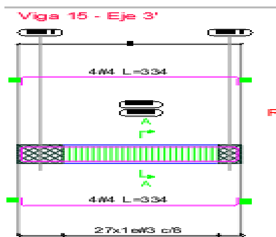
Ilustración 42. Disposición de refuerzo viga 3*(B-E) N +15.40
