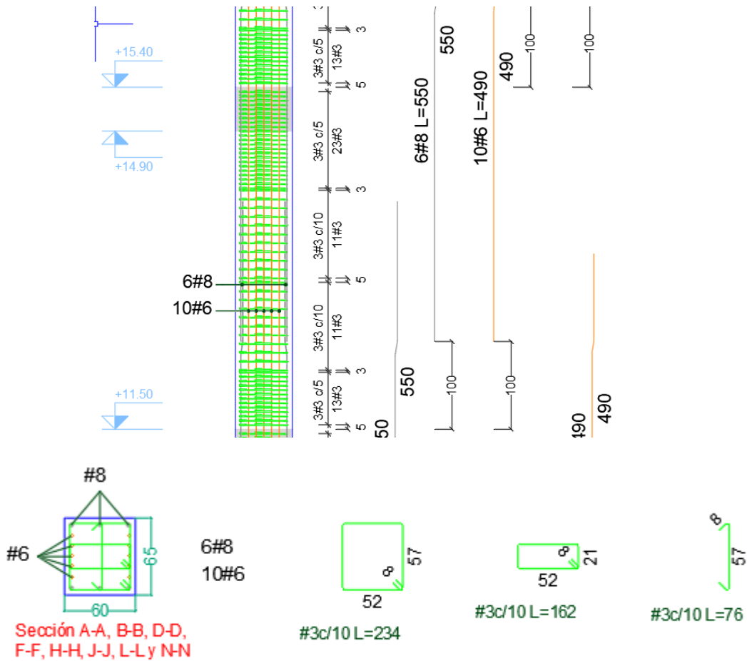
Ilustración 4. Disposición acero de refuerzo columna C3.
