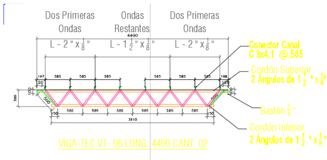
Ilustración 22. Detalle joist VT 06.
