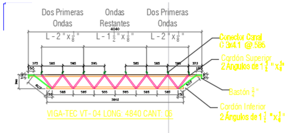
Ilustración 20. Detalle joist VT 04
