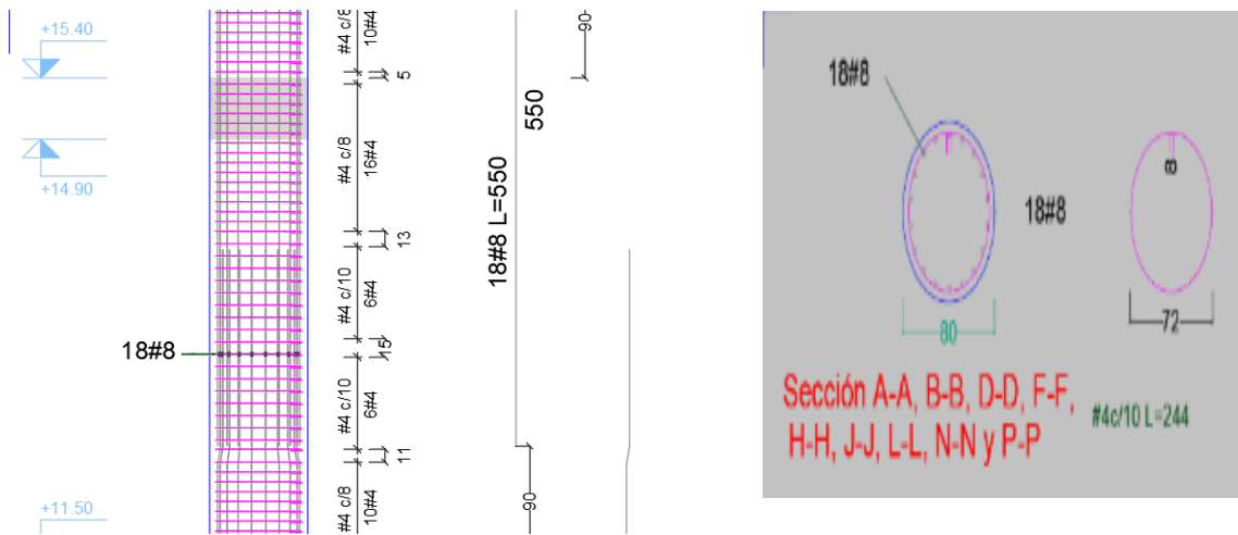
Ilustración 2. Disposición acero de refuerzo columna C1.
