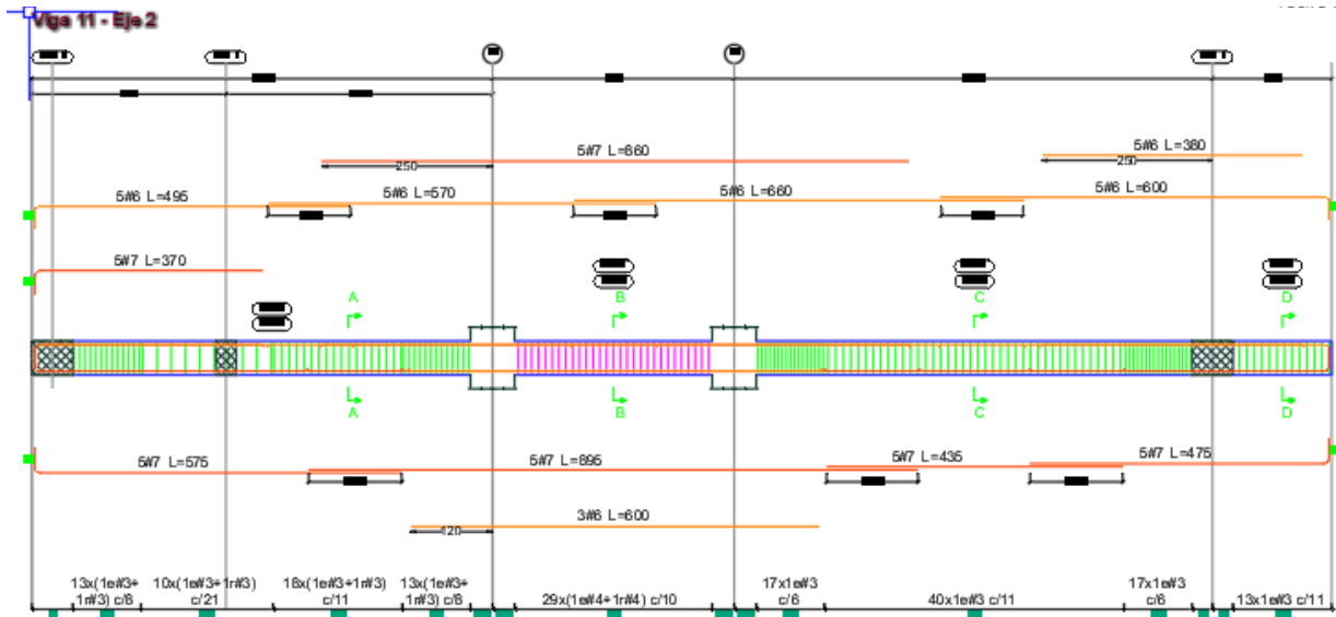
Ilustración 40. Disposición de refuerzo viga 2 (B-E) N +19.30
