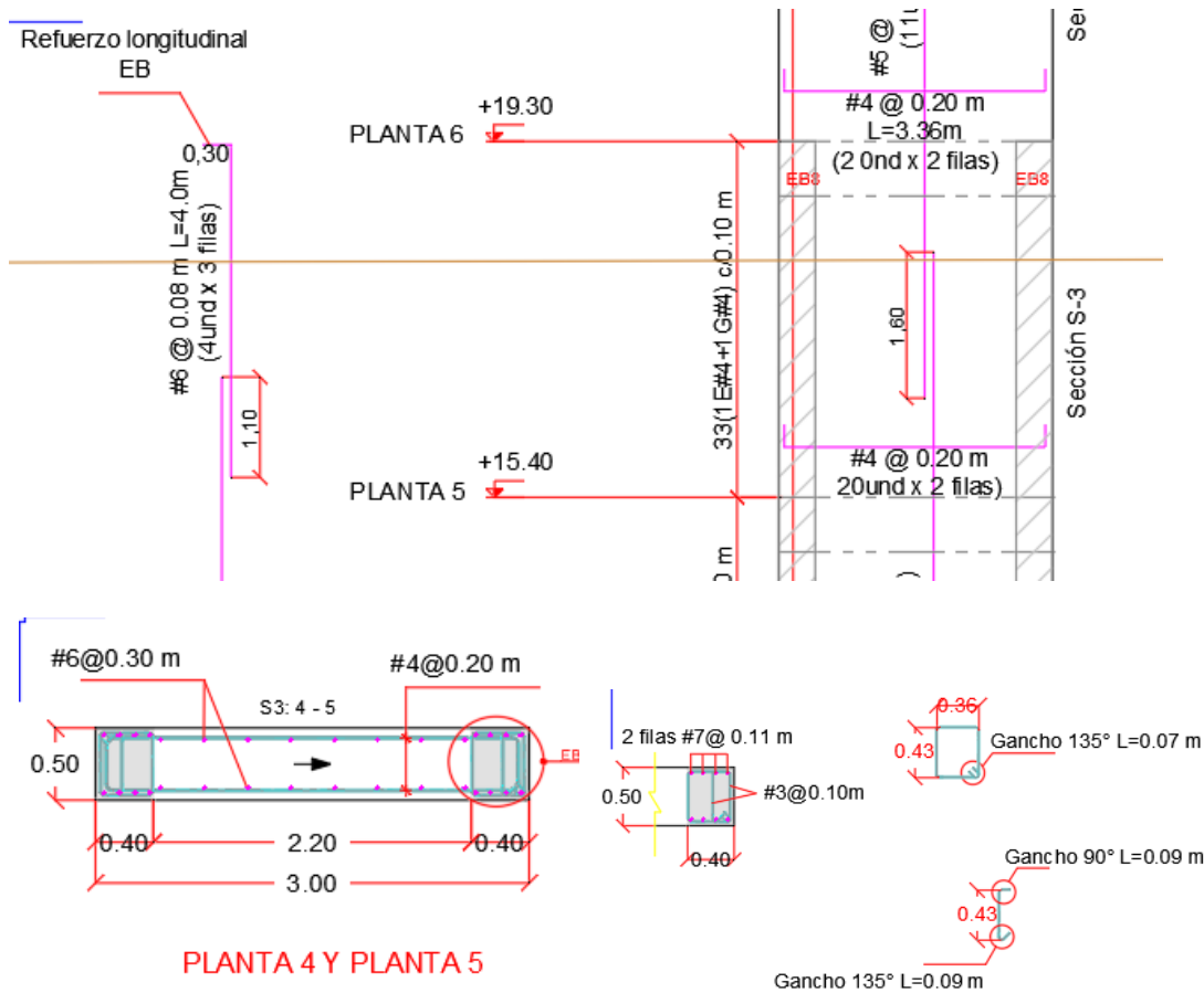
Ilustración 10. Disposición acero de refuerzo pantalla PW4.
