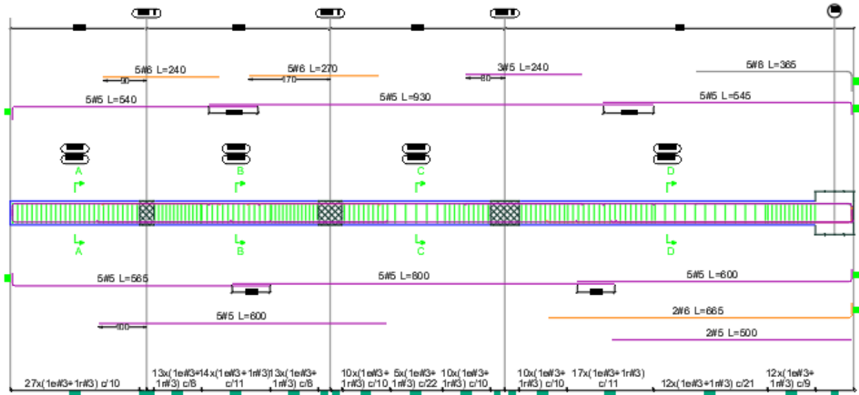
Ilustración 43. Disposición de refuerzo viga 4 (B-E) N +19.30
