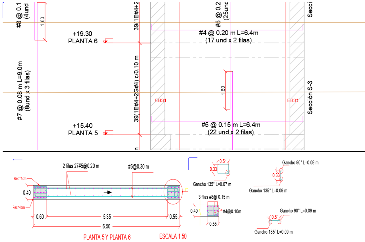
Ilustración 16. Disposición acero de refuerzo pantalla PW10.
