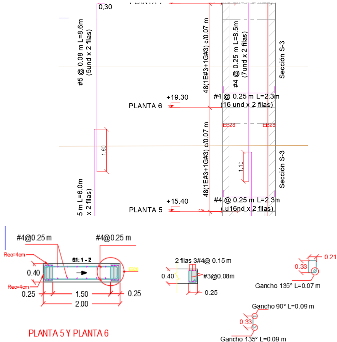
Ilustración 11. Disposición acero de refuerzo pantalla PW5.
