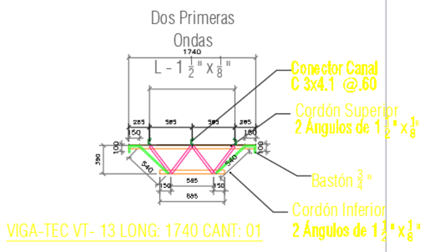
Ilustración 29. Detalle joist VT 13
