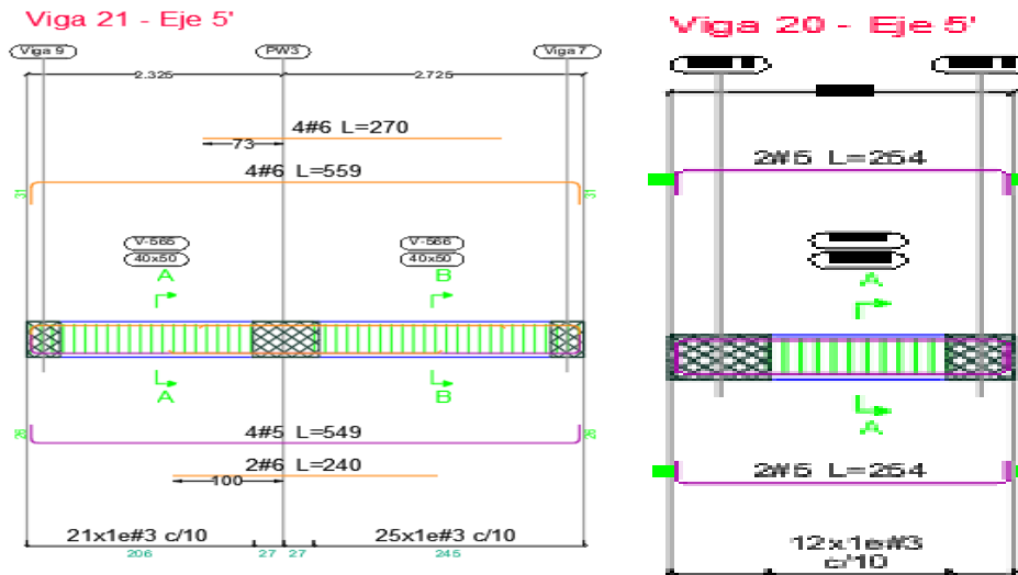
Ilustración 46. Disposición de refuerzo viga 5' (B-E) N +19.30
