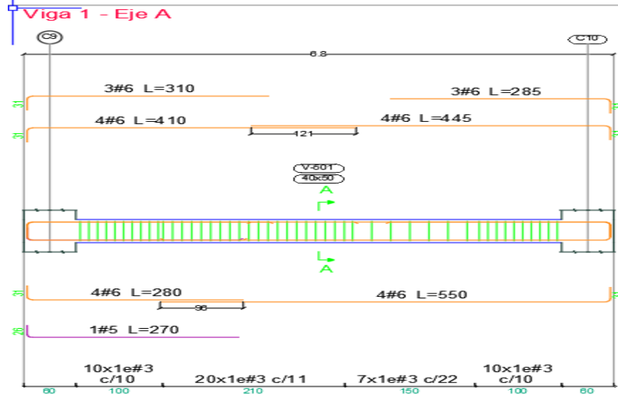
Ilustración 32. Disposición de refuerzo viga A' N+19.30
