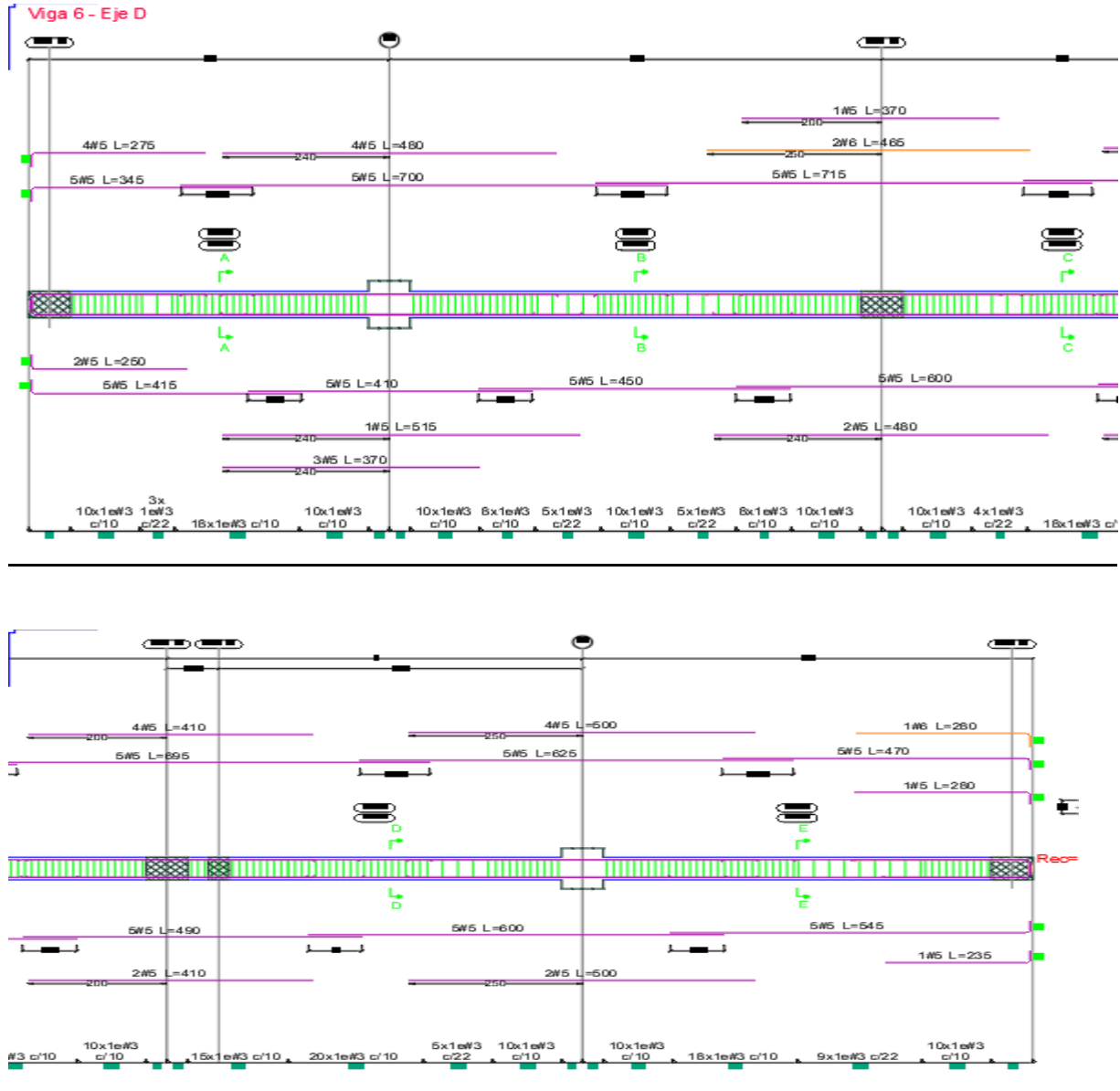
Ilustración 35. Disposición de refuerzo viga D (1'-2) N +15.40
