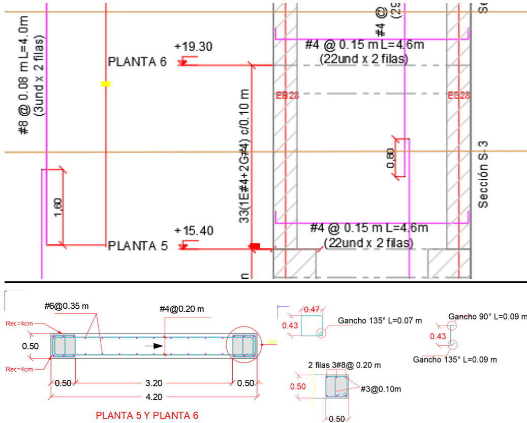
Ilustración 15. Disposición acero de refuerzo pantalla PW9.
