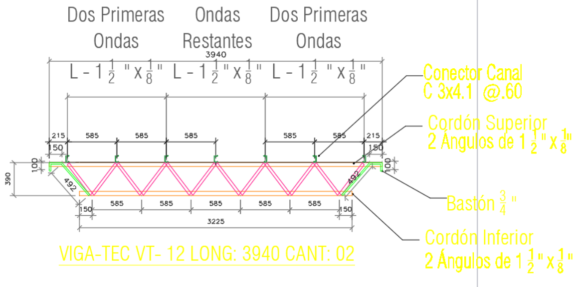
Ilustración 28. Detalle joist VT 12
