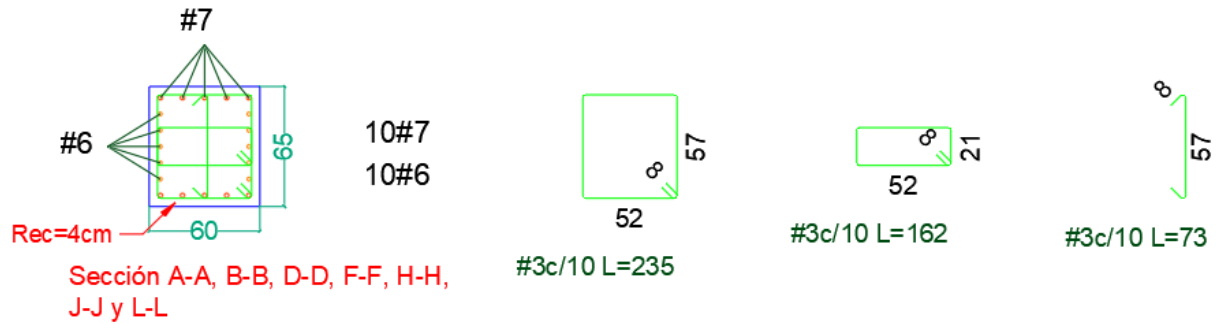
Ilustración 3. Disposición acero de refuerzo columna C2, C4 y C5
