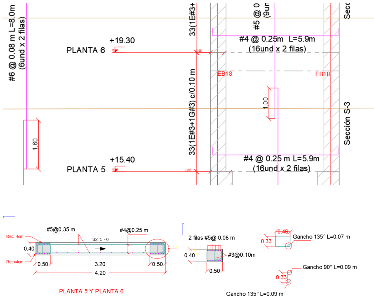
Ilustración 12. Disposición acero de refuerzo pantalla PW6.
