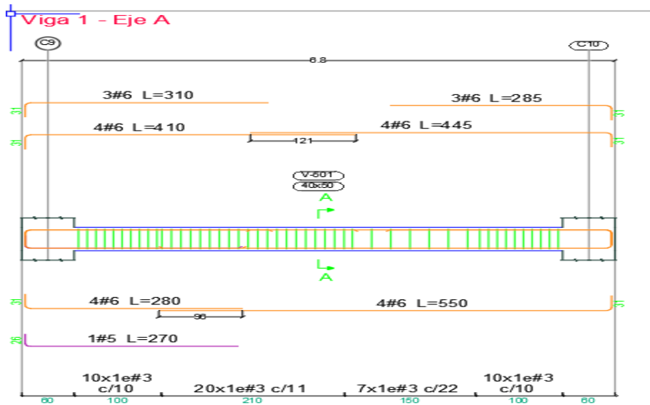
Ilustración 31. Disposición de refuerzo viga A N +19.30.
