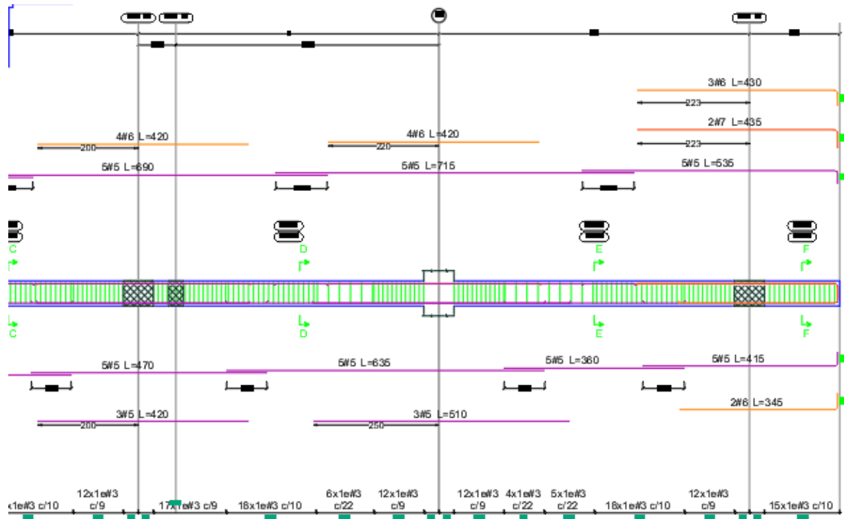
Ilustración 34. Disposición de refuerzo viga C N +15.40.
