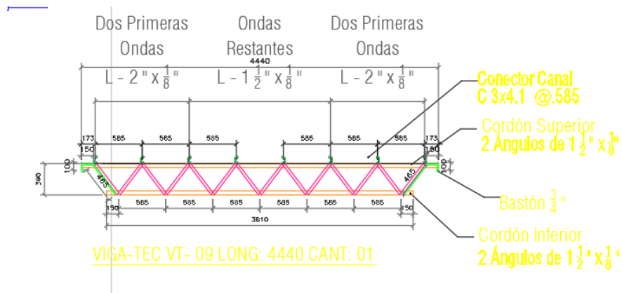
Ilustración 25. Detalle joist VT 09
