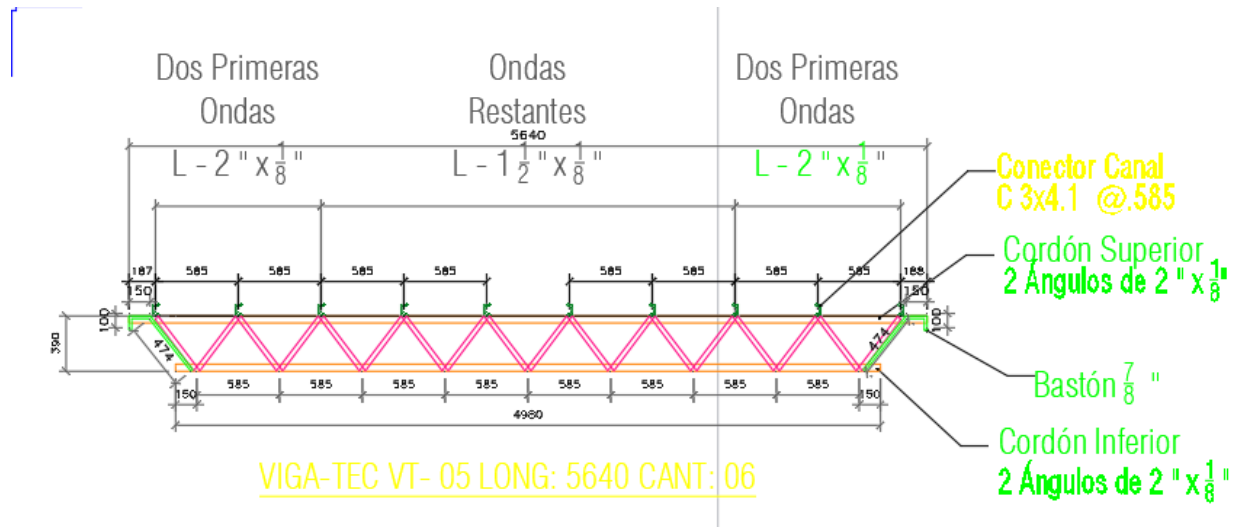
Ilustración 21. Detalle joist VT 05.
