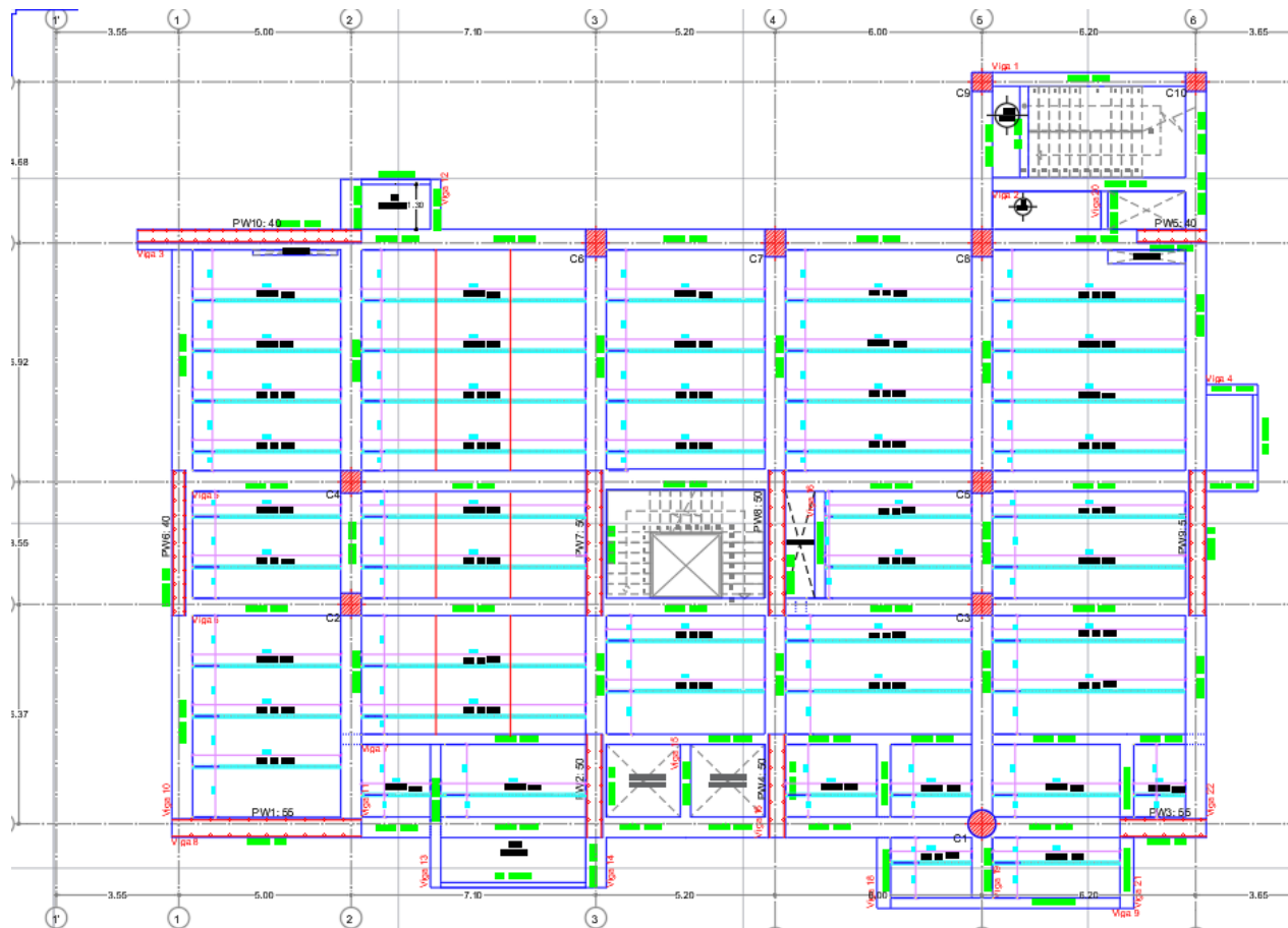
Ilustración 30. Disposición de vigas joist entrepiso 5 N+19.30
