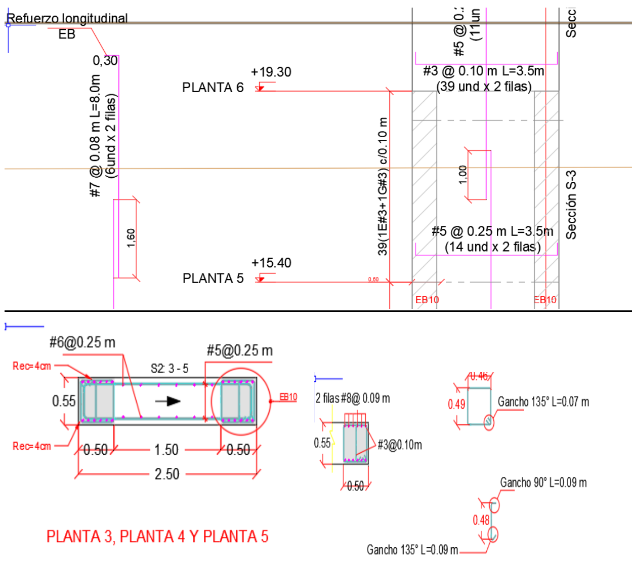
Ilustración 9. Disposición acero de refuerzo pantalla PW3.
