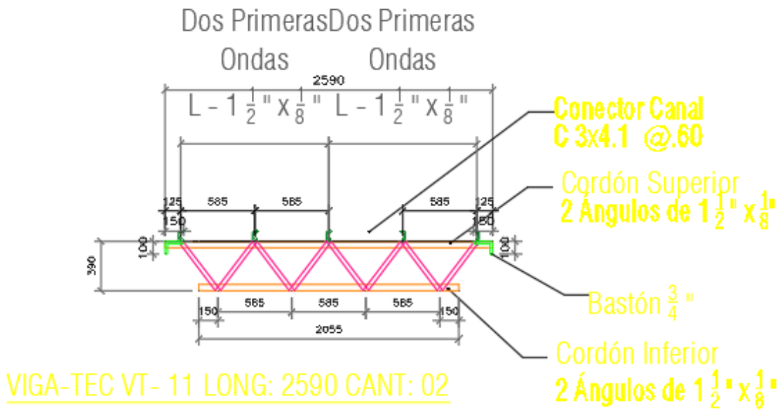
Ilustración 27. Detalle joist VT 11
