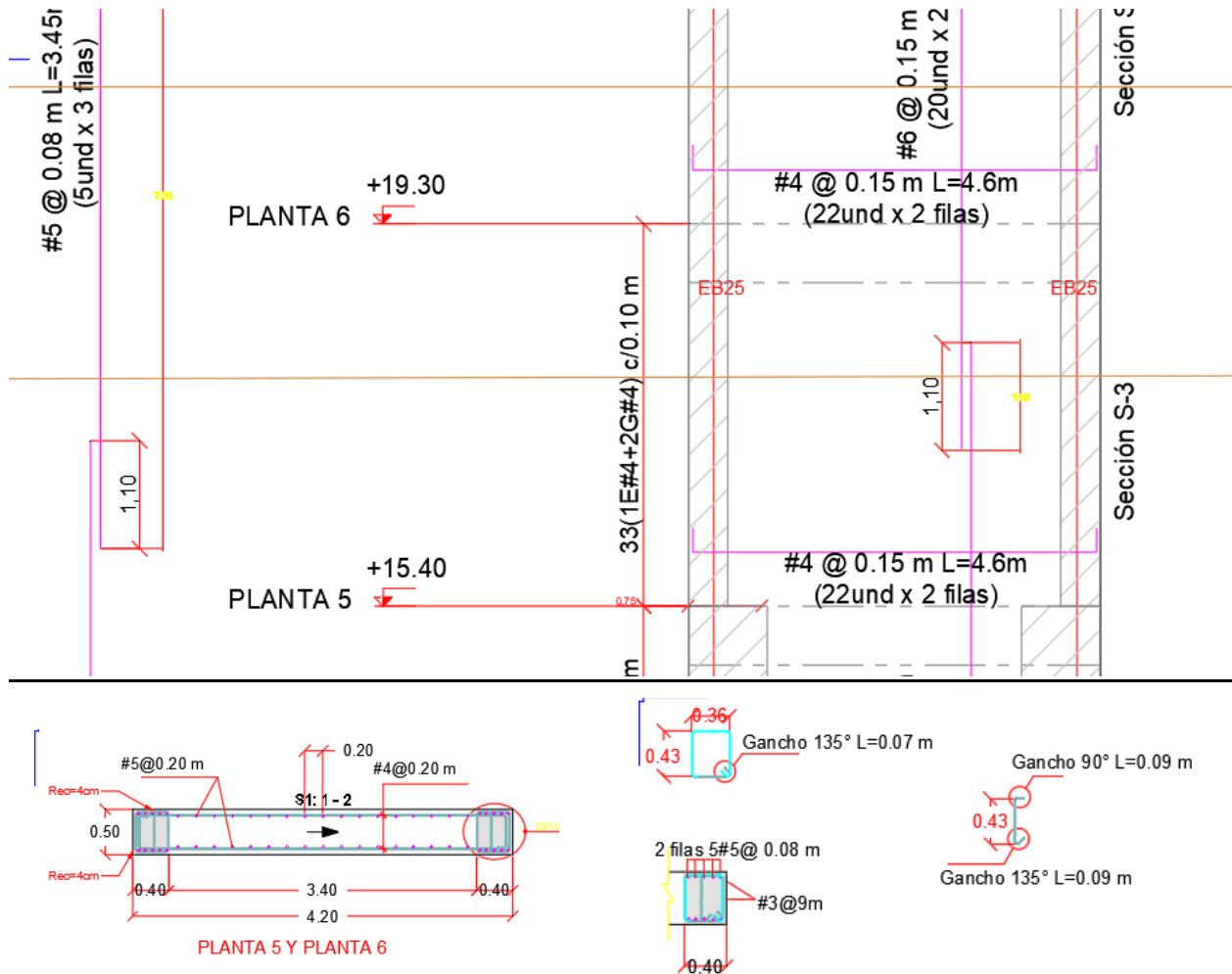
Ilustración 14. Disposición acero de refuerzo pantalla PW8.
