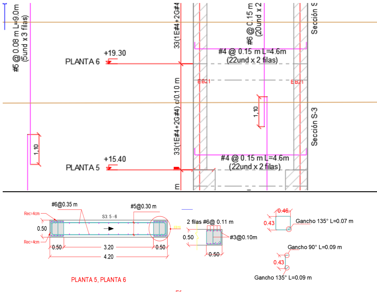
Ilustración 13. Disposición acero de refuerzo pantalla PW7.
