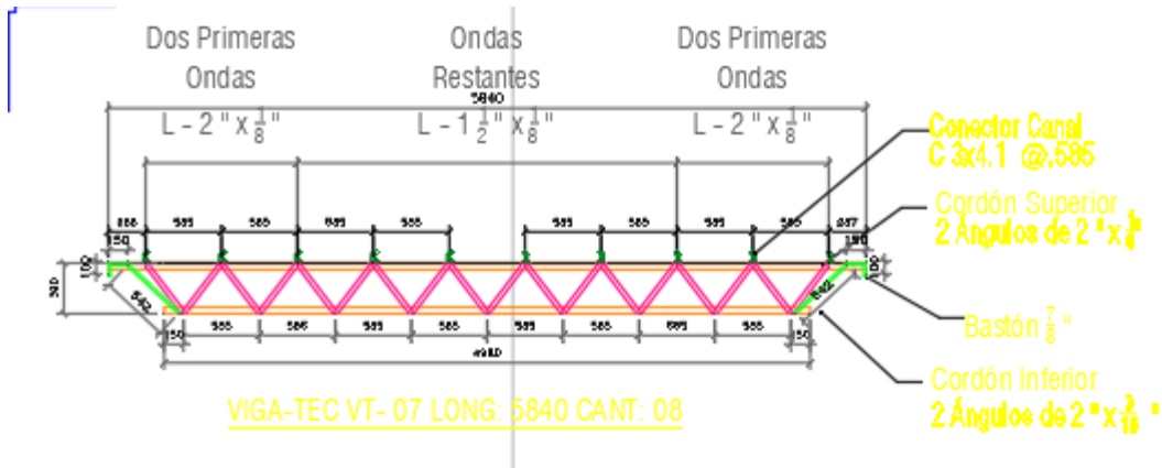
Ilustración 23. Detalle joist VT 07.
