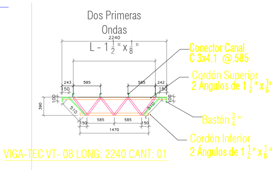
Ilustración 24. Detalle joist VT 08
