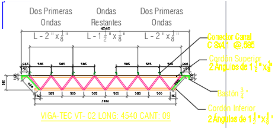
Ilustración 18. Detalle joist VT 02
