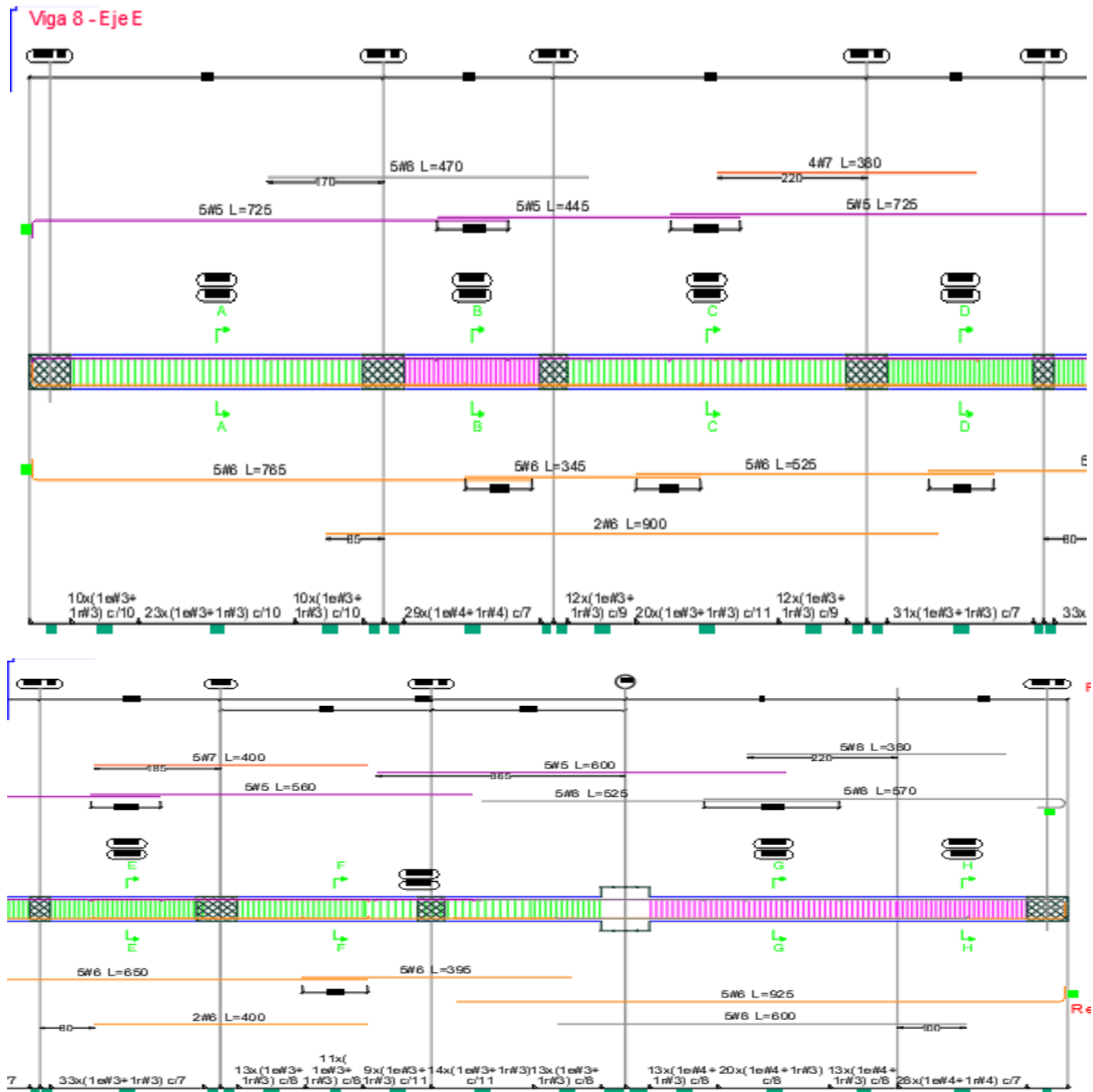
Ilustración 37. Disposición de refuerzo viga E (1-6) N + 19.30
