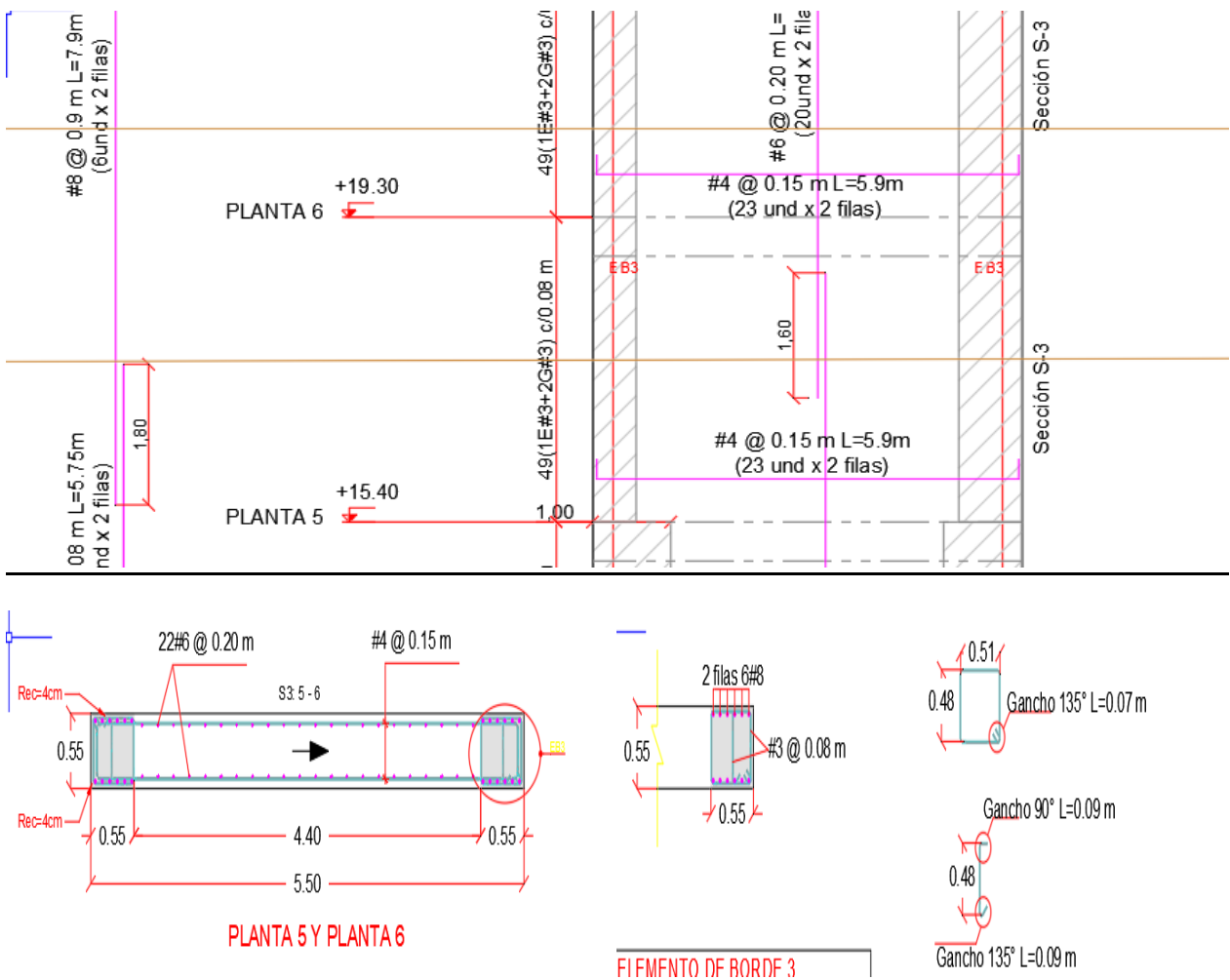
Ilustración 7. Disposición acero de refuerzo pantalla PW1.
