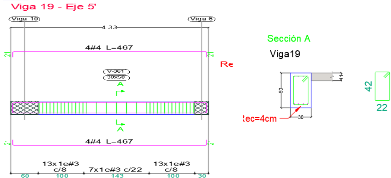
Ilustración 48. Disposición de refuerzo viga 5' (B-E) N +15.40
