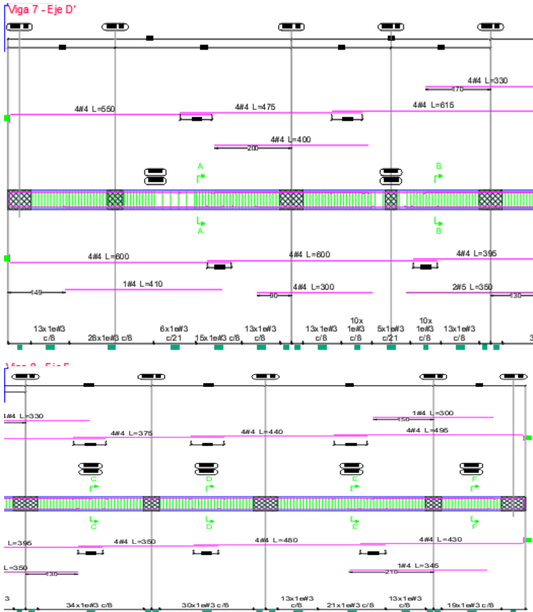
Ilustración 36. Disposición de refuerzo viga D (1'-6') N +15.40.
