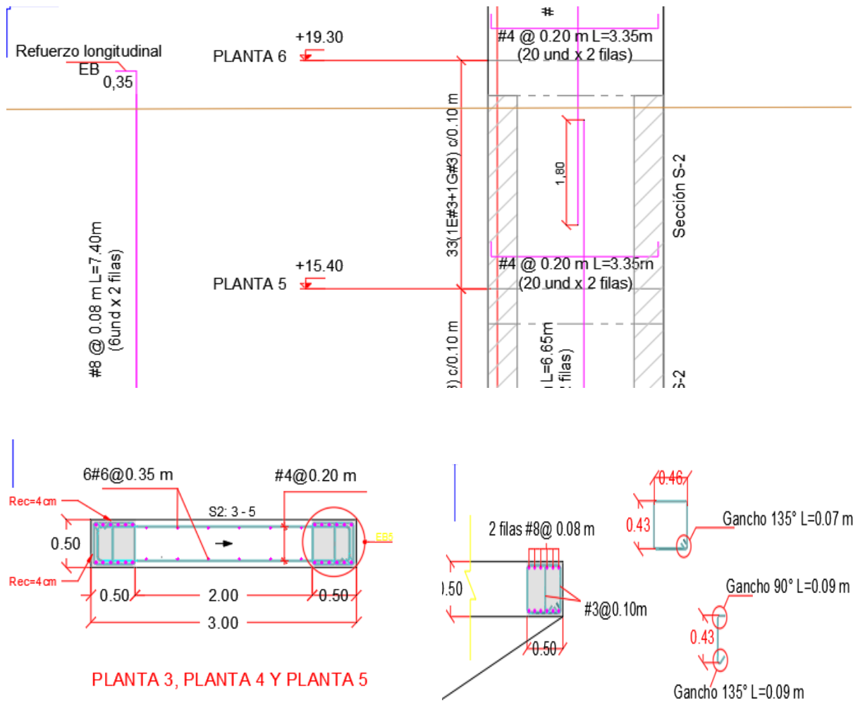
Ilustración 8. Disposición acero de refuerzo pantalla PW2
