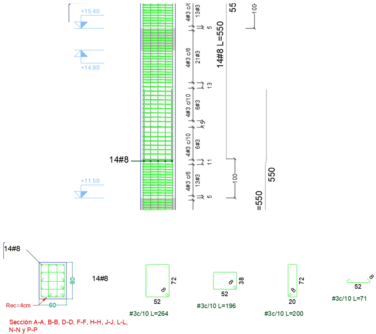
Ilustración 5. Disposición acero de refuerzo columna C6, C7 y C8.
