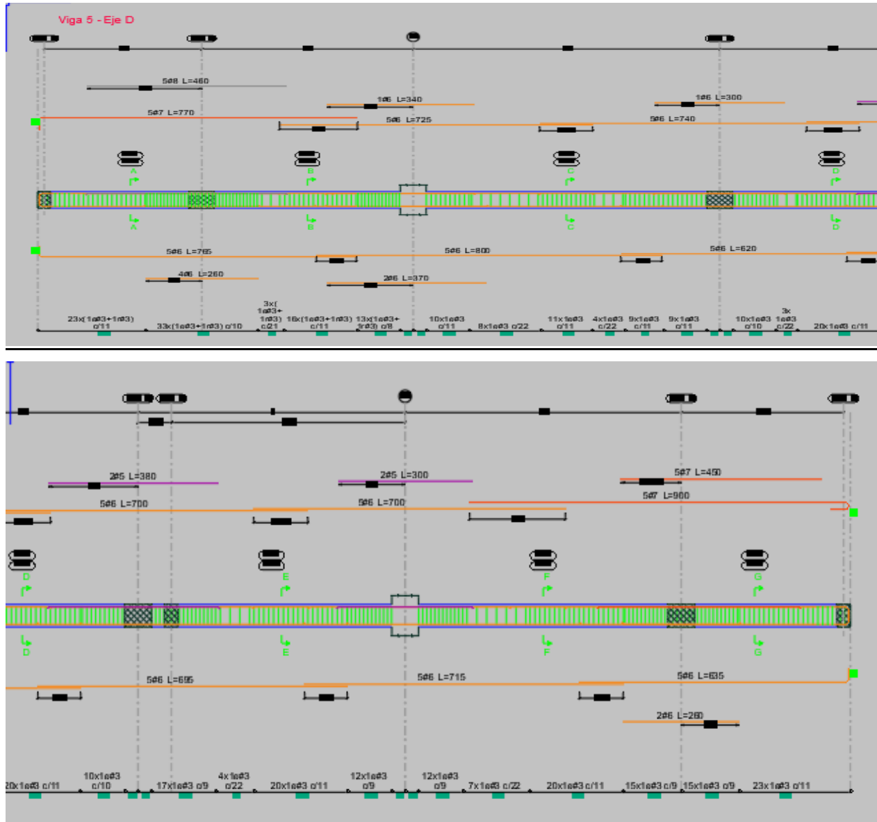
Ilustración 33. Disposición de refuerzo viga D (1'-2) N +11.50
