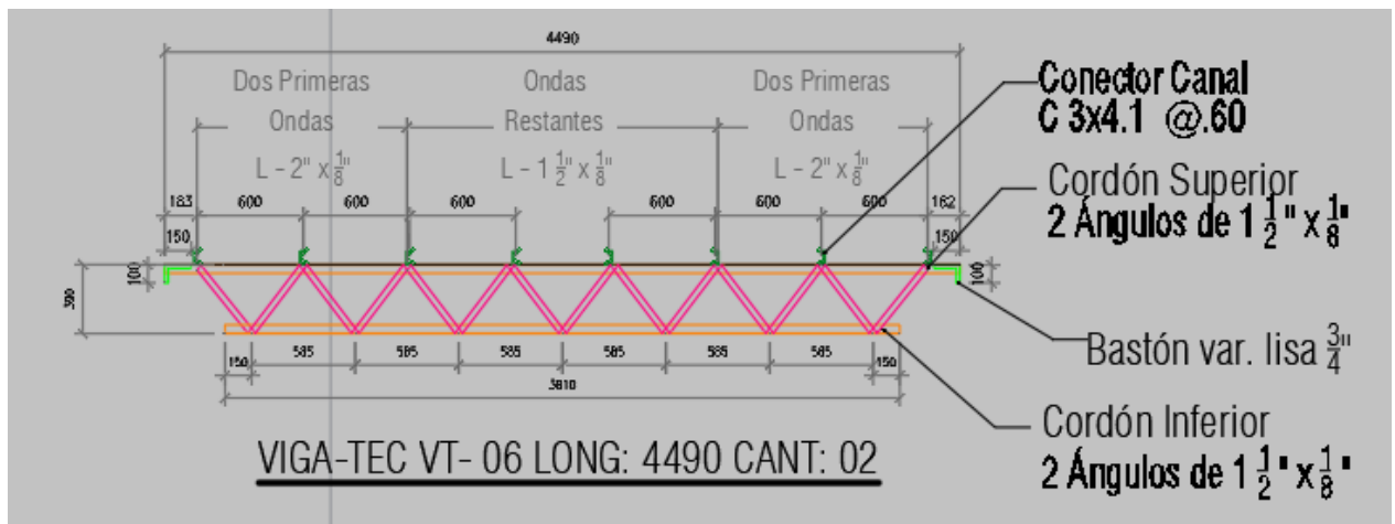
Ilustración 24. Detalle joist VT 06.
