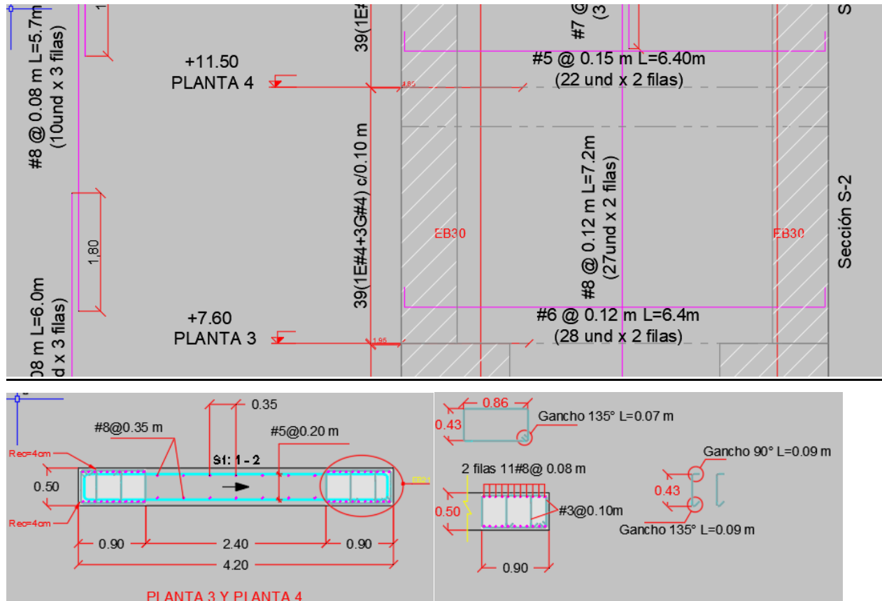
Ilustración 16. Disposición acero de refuerzo pantalla PW9.
