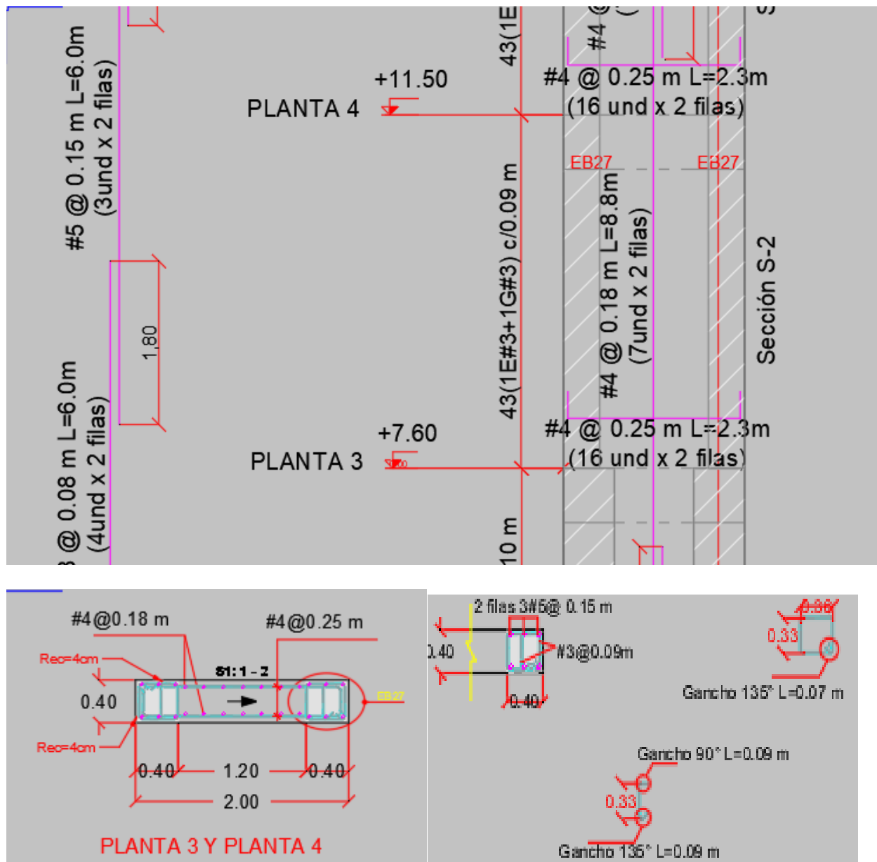
Ilustración 12. Disposición acero de refuerzo pantalla PW5.
