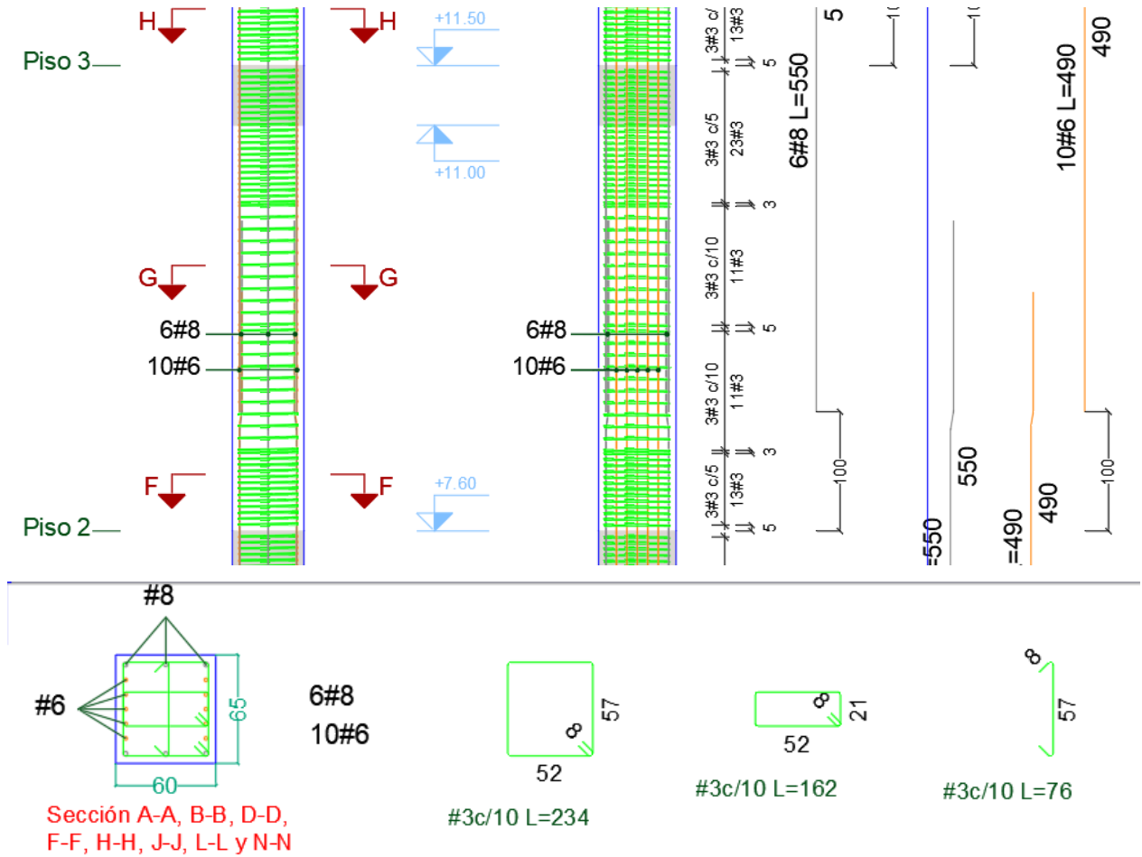
Ilustración 5. Disposición acero de refuerzo columna C3.
