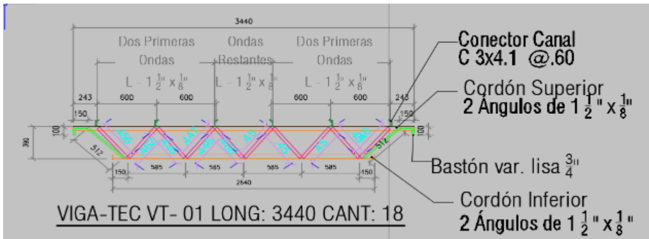
Ilustración 19. Detalle joist VT 01
