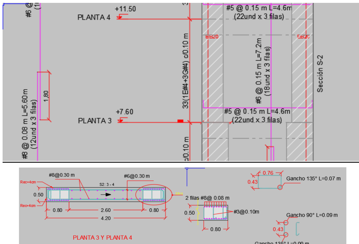
Ilustración 14. Disposición acero de refuerzo pantalla PW7.
