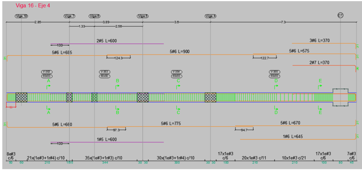
Ilustración 41. Disposición de refuerzo viga 4 (B-E) N +11.50
