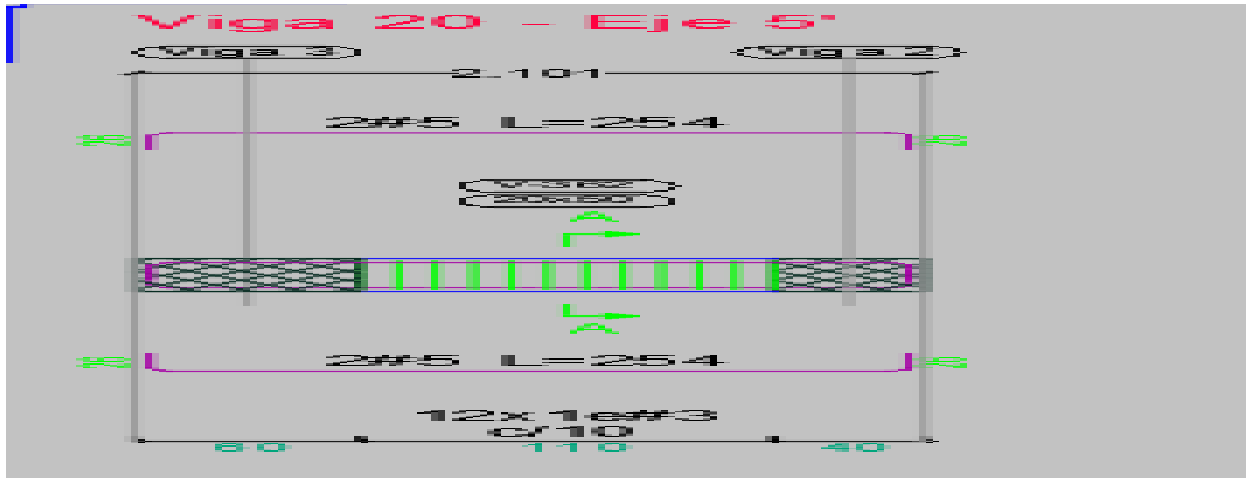
Ilustración 45. Disposición de refuerzo viga 5' ' (B-E) N +11.50
