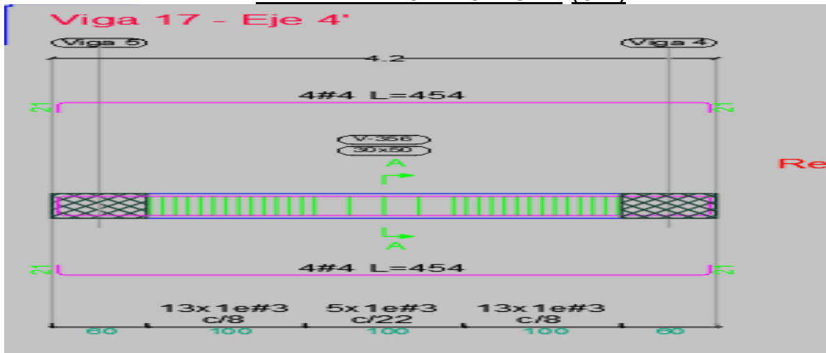
Ilustración 42. Disposición de refuerzo viga 4' (C-D) N +11.50
