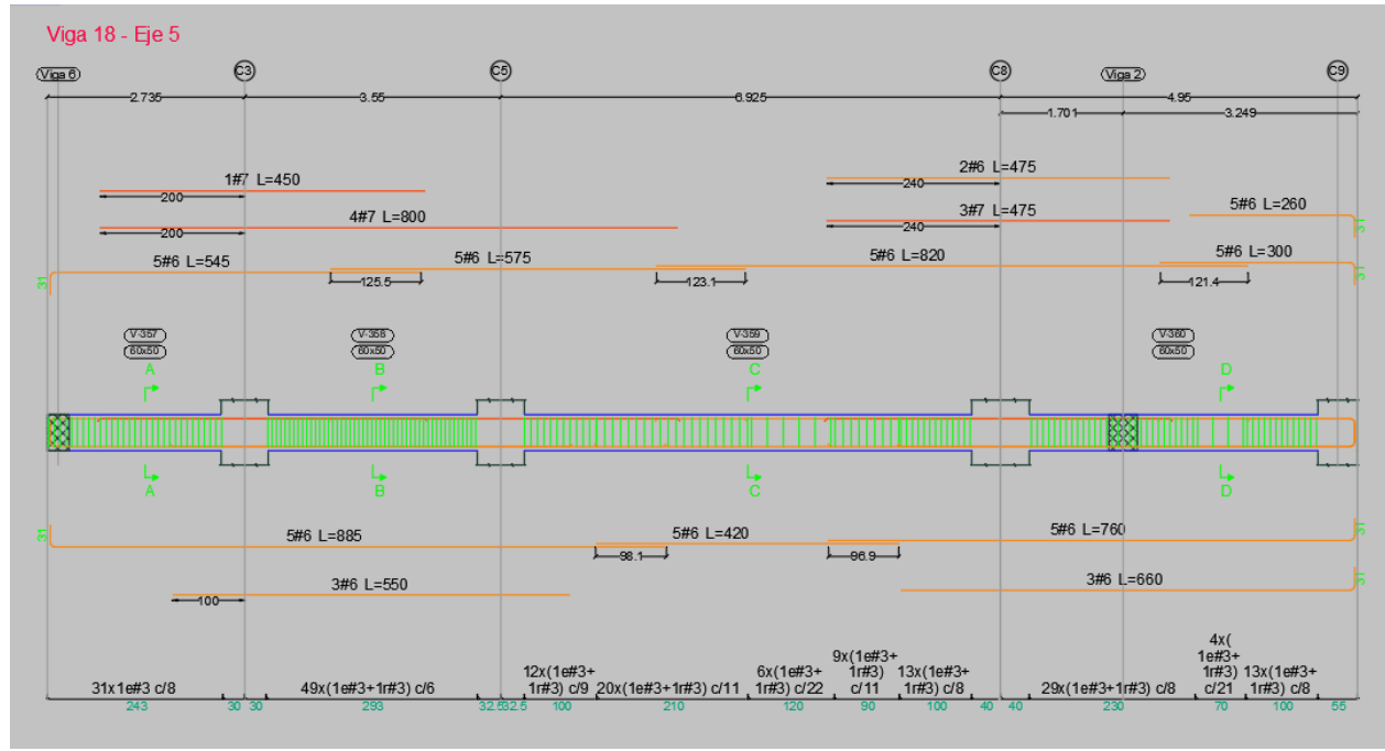
Ilustración 43. Disposición de refuerzo viga 5 (B-E) N +11.50
