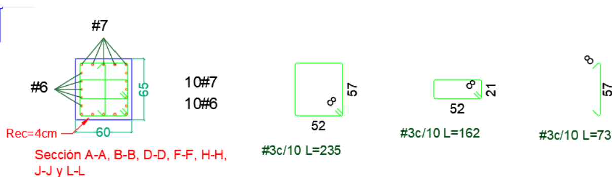
Ilustración 4. Disposición acero de refuerzo columna C2, C4 y C5
