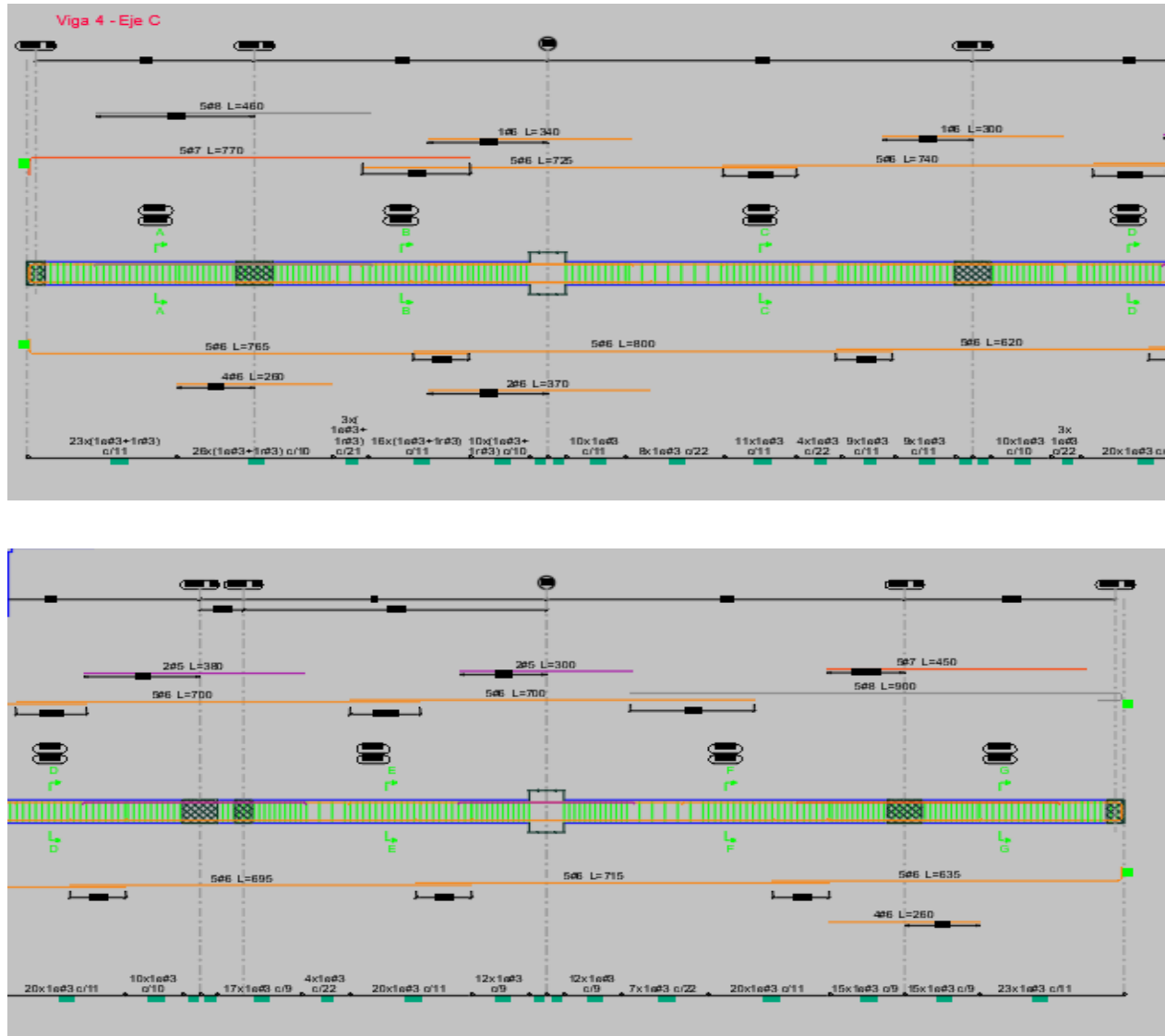
Ilustración 32. Disposición de refuerzo viga C N +11.50.
