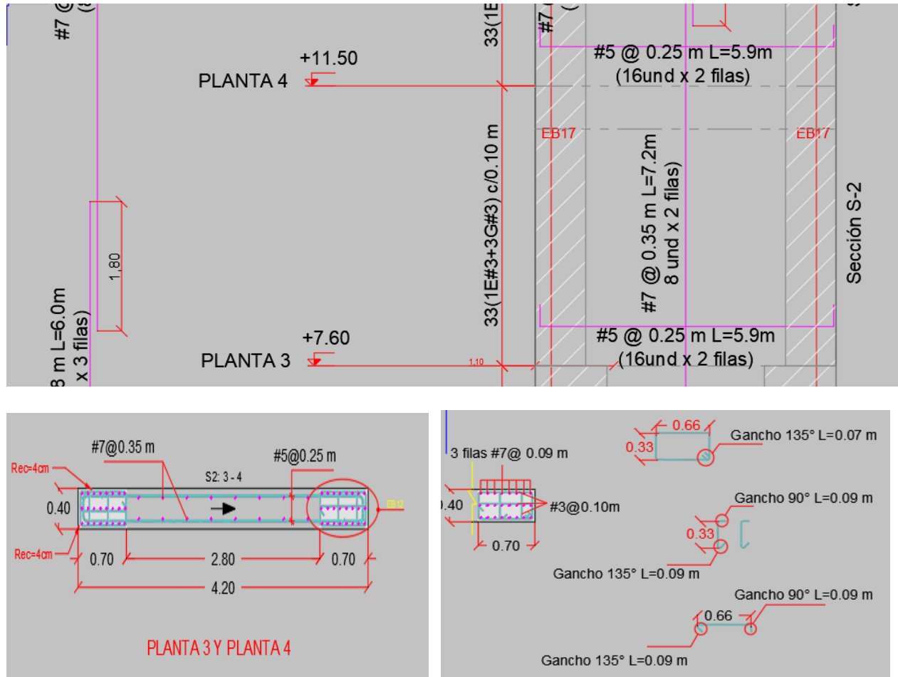
Ilustración 13. Disposición acero de refuerzo pantalla PW6.
