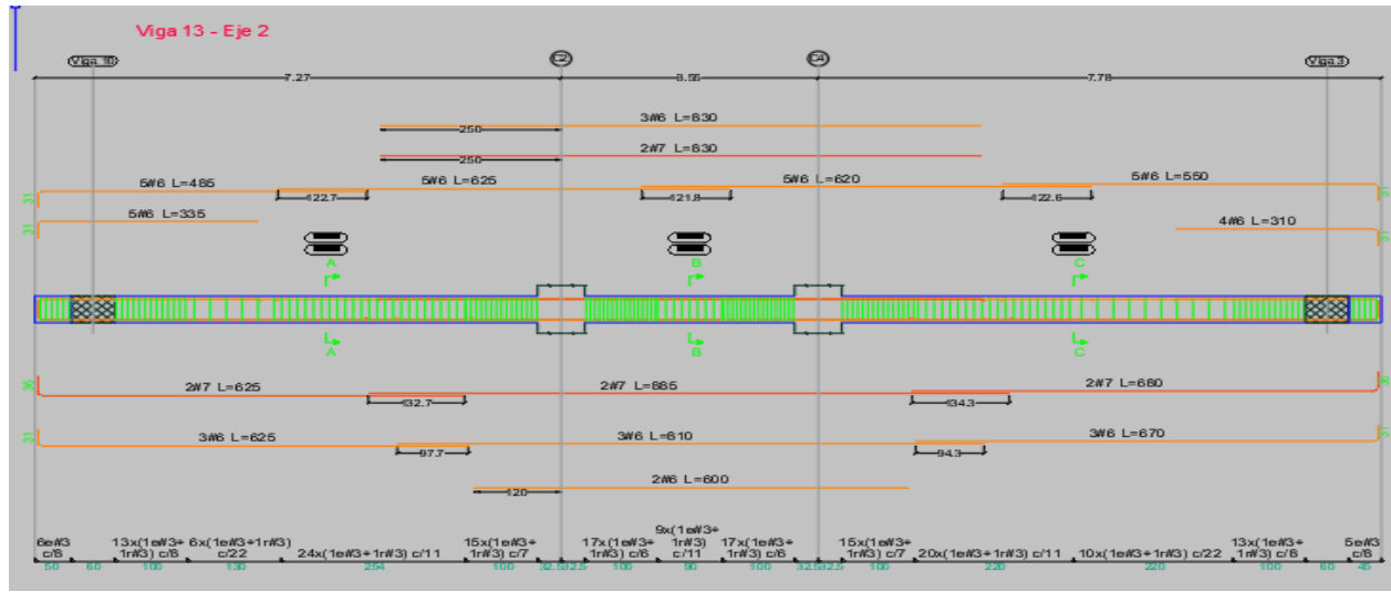
Ilustración 38. Disposición de refuerzo viga 2 (B-E) N +11.50
