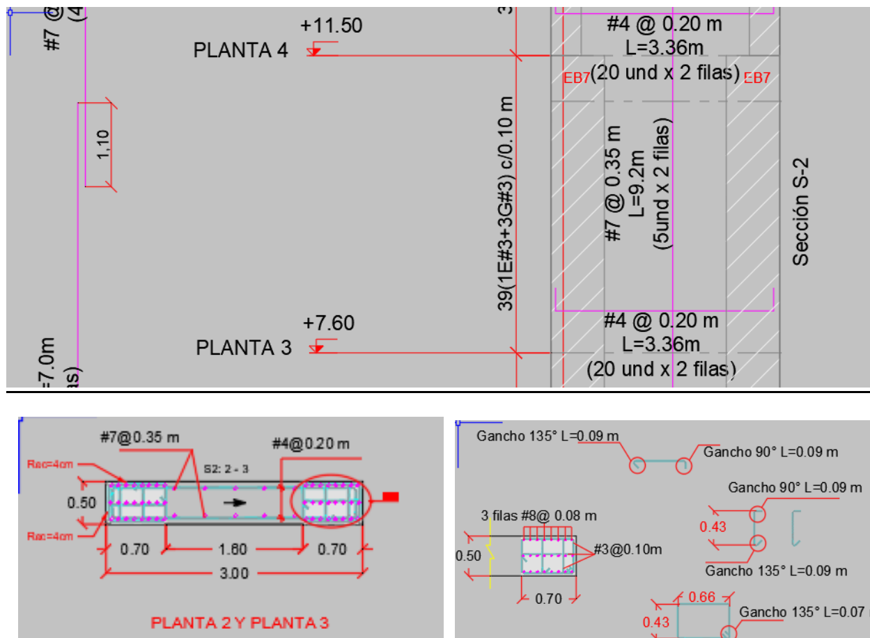
Ilustración 11. Disposición acero de refuerzo pantalla PW4.
