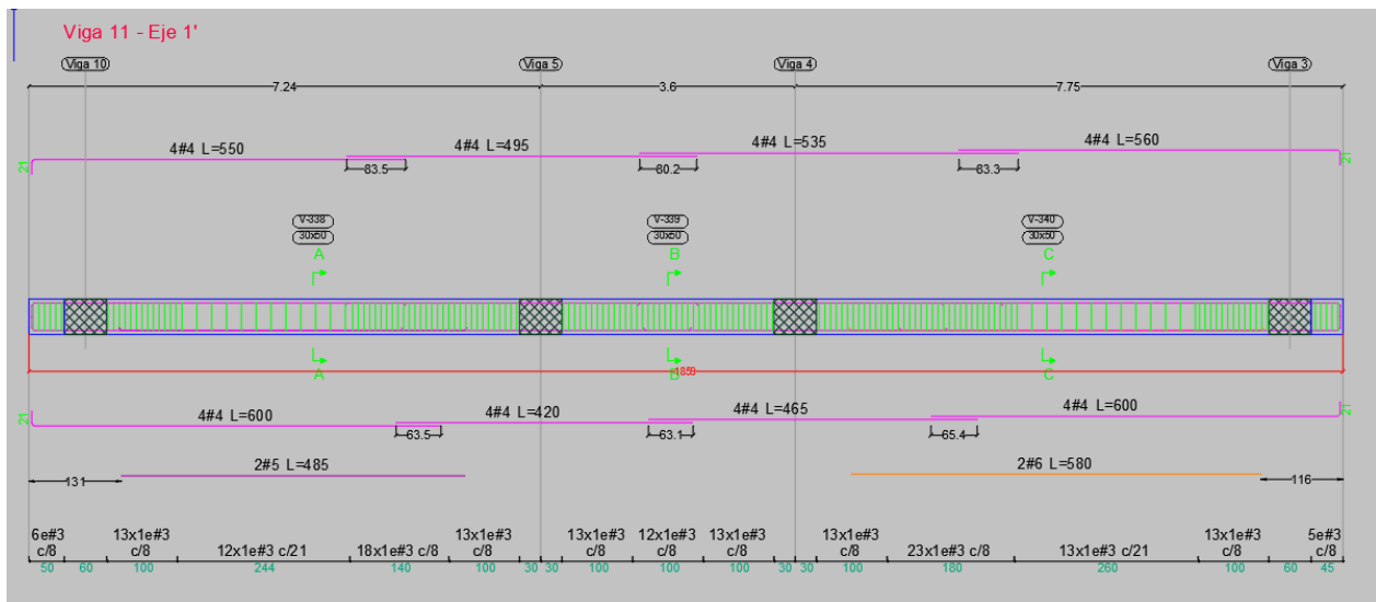
Ilustración 36. Disposición de refuerzo viga 1' (B-E) N +11.50
