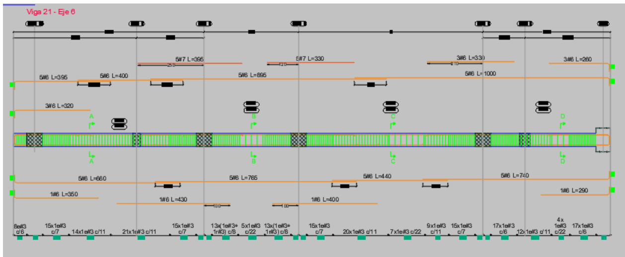
Ilustración 46. Disposición de refuerzo viga 6 (A-E) N +11.50
