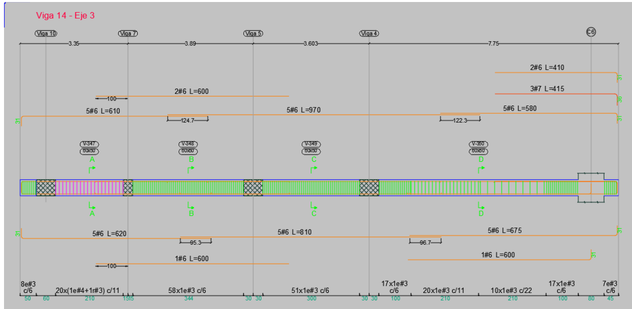
Ilustración 39. Disposición de refuerzo viga 3 (B-E) N +11.50
