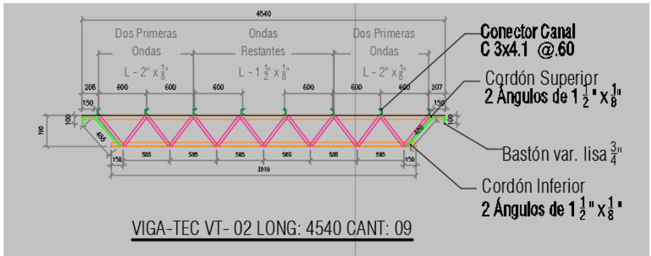
Ilustración 20. Detalle joist VT 02.
