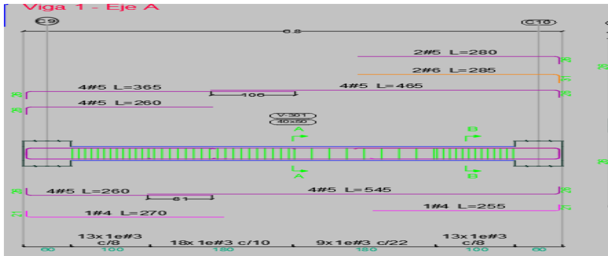
Ilustración 29. Disposición de refuerzo viga A N +11.50.
