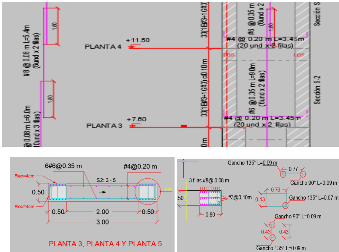
Ilustración 9. Disposición acero de refuerzo pantalla PW2
