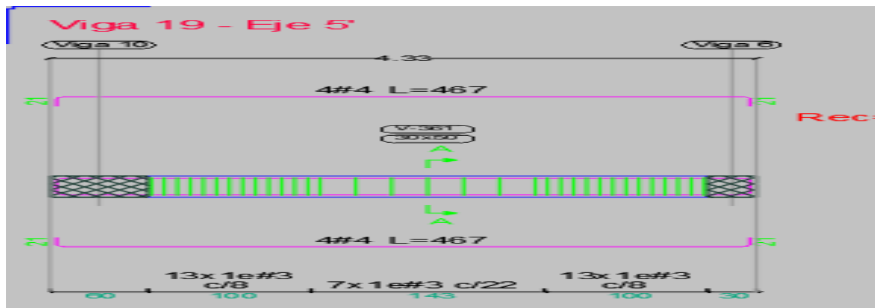
Ilustración 44. Disposición de refuerzo viga 5' (B-E) N +11.50
