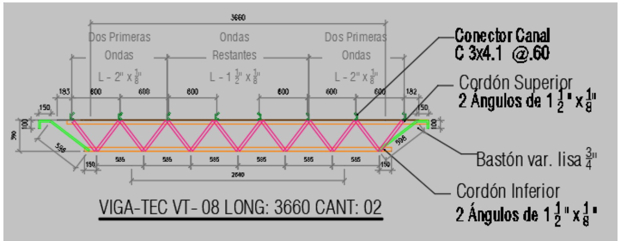
Ilustración 26. Detalle joist VT 08
