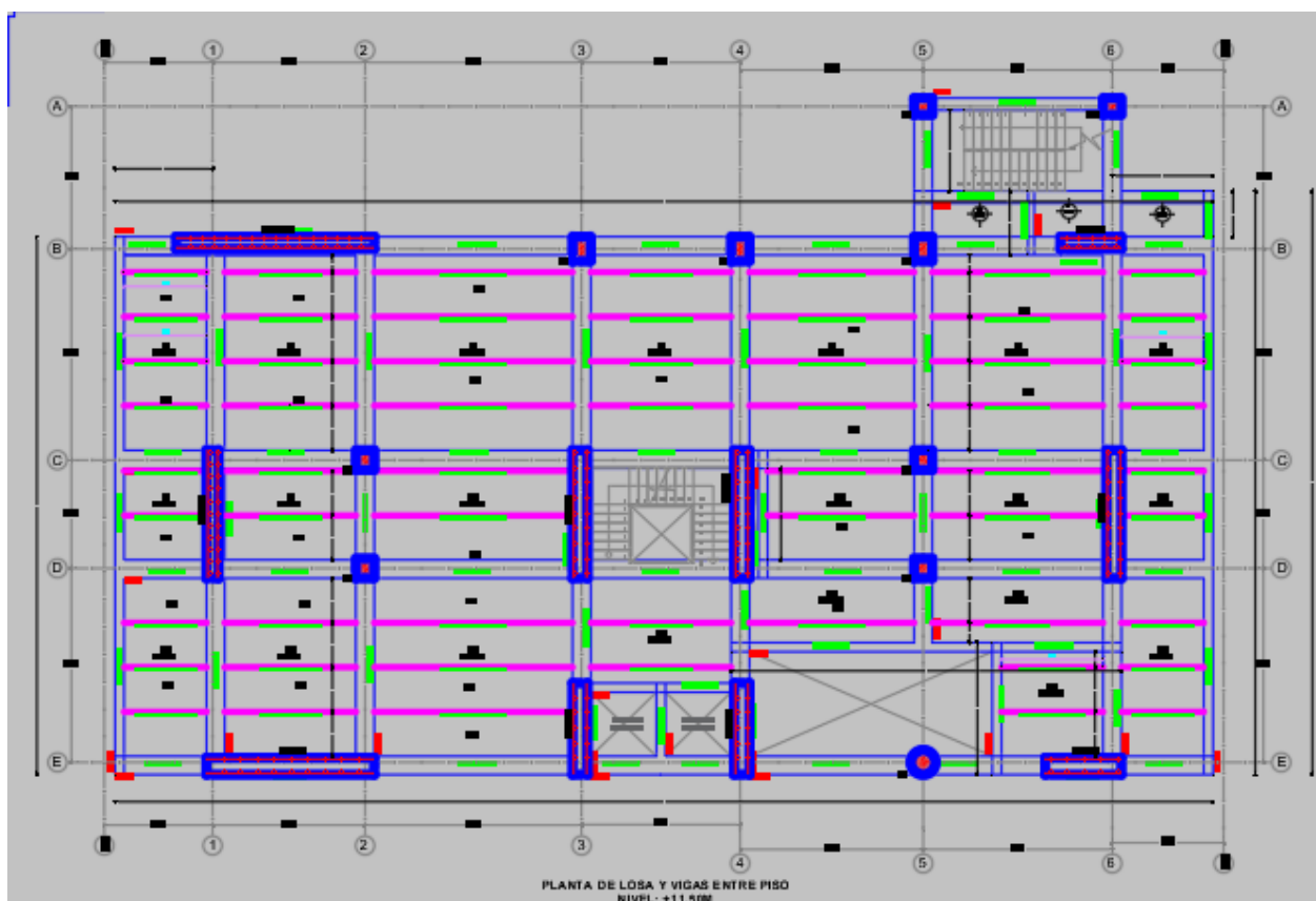
Ilustración 28. Disposición de vigas joist
