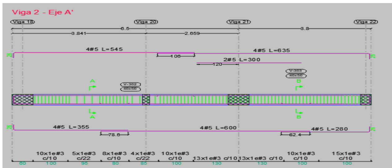
Ilustración 30. Disposición de refuerzo viga A' N +11.50
