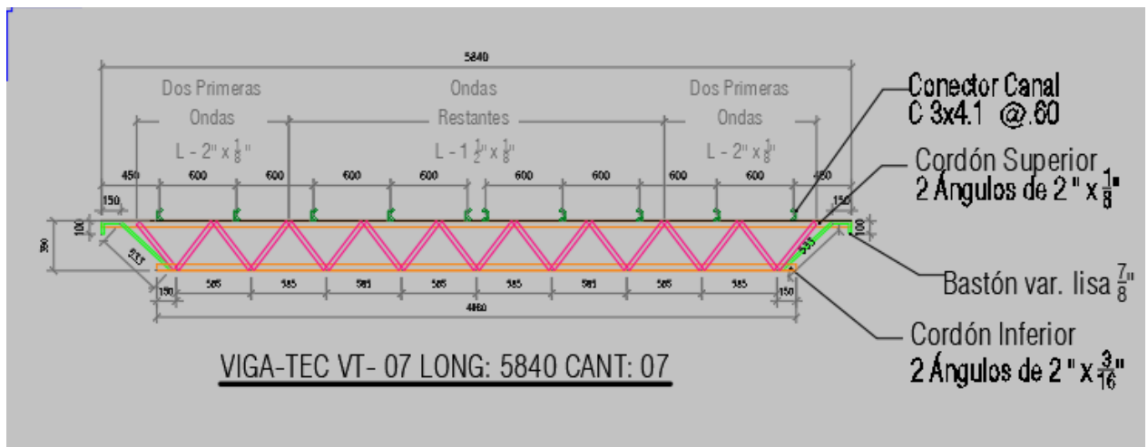
Ilustración 25. Detalle joist VT 07.
