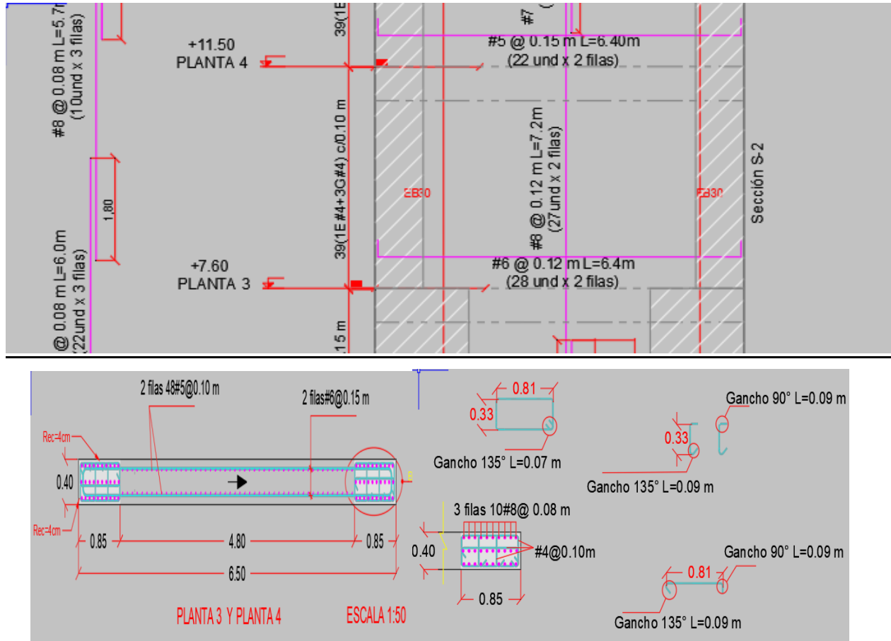
Ilustración 17. Disposición acero de refuerzo pantalla PW10.
