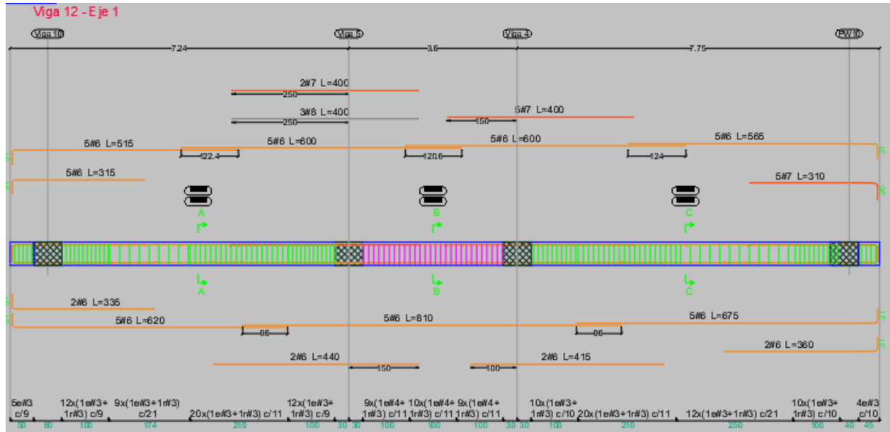
Ilustración 37. Disposición de refuerzo viga 1 (B-E) N +11.50
