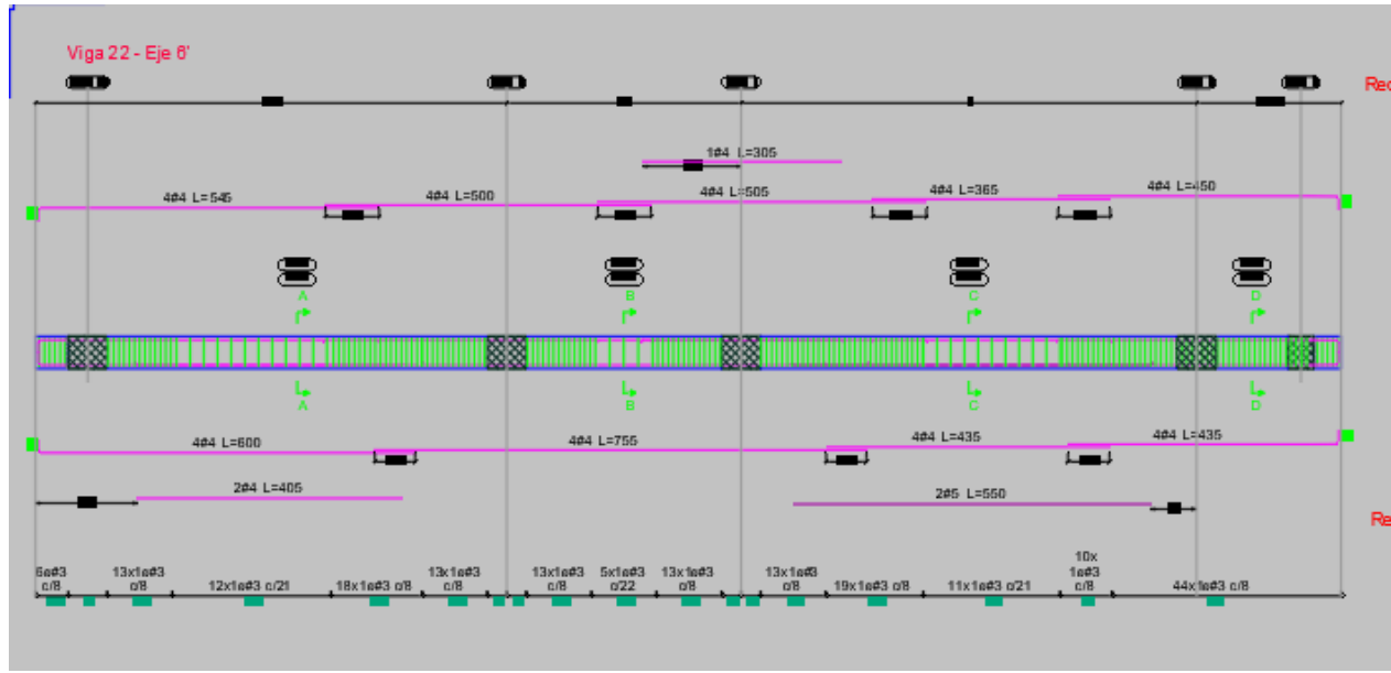
Ilustración 47. Disposición de refuerzo viga 6' (A-E) N +11.50
