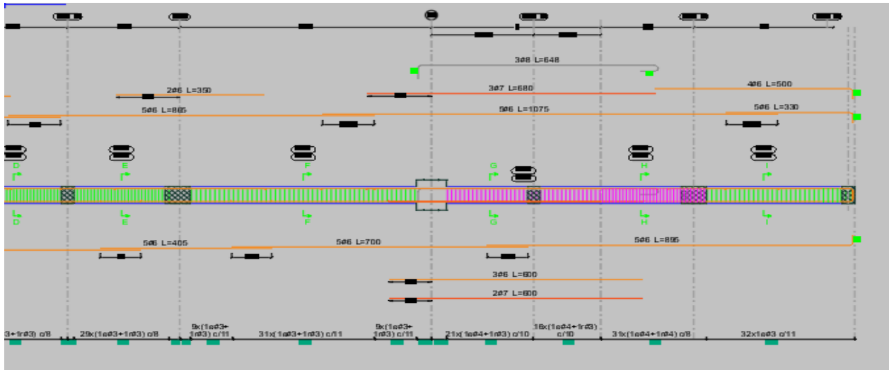
Ilustración 35. Disposición de refuerzo viga E (1'-6') N +11.50
