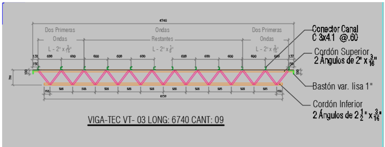
Ilustración 21. Detalle joist VT 03.
