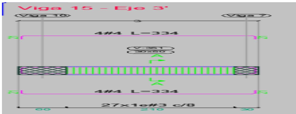
Ilustración 40. Disposición de refuerzo viga 3' (B-E) N +11.50
