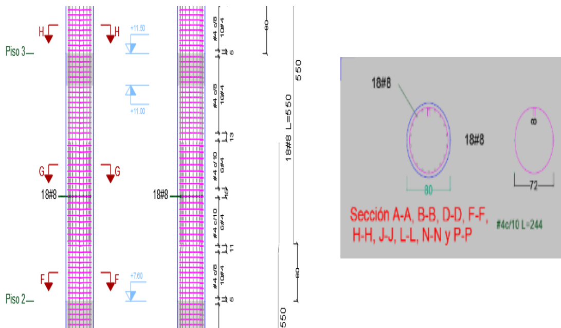
Ilustración 3. Disposición acero de refuerzo columna C1
