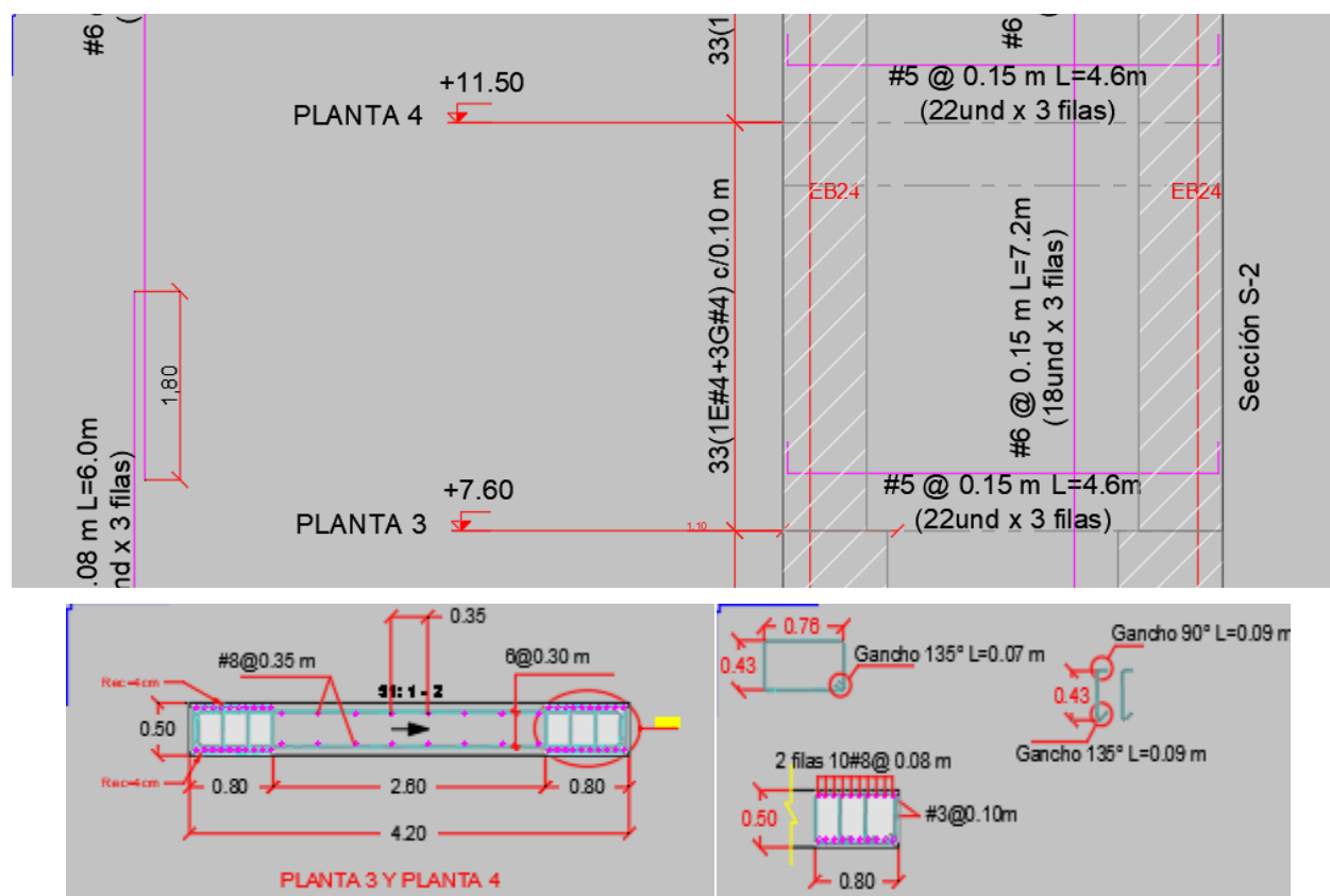
Ilustración 15. Disposición acero de refuerzo pantalla PW8.
