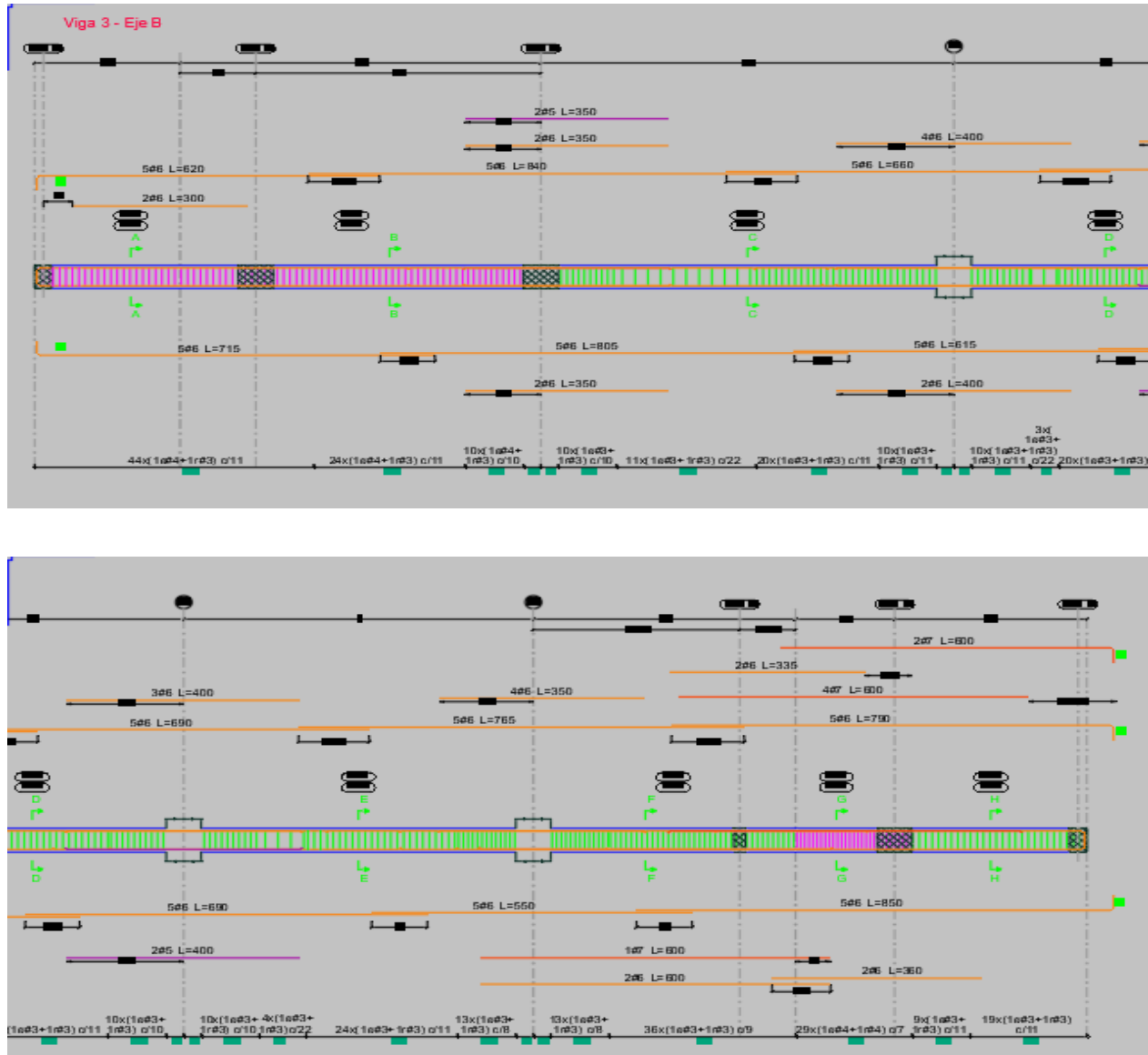
Ilustración 31. Disposición de refuerzo viga B N +11.50.
