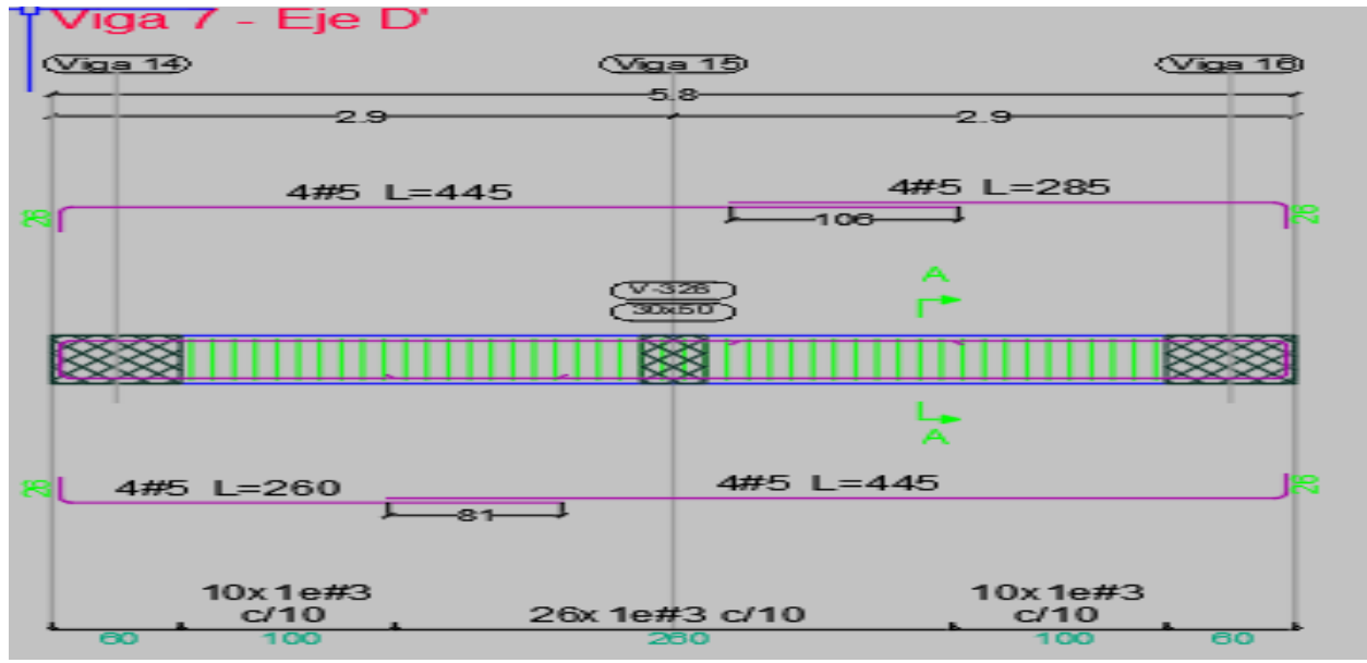
Ilustración 34. Disposición de refuerzo viga D (1'-6') N +11.50.
