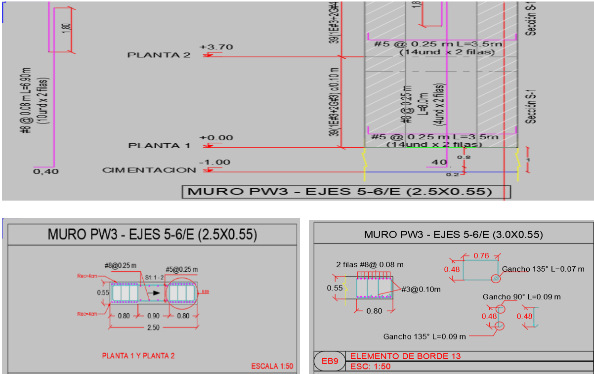
Ilustración 14. Disposición refuerzo pantalla PW3
