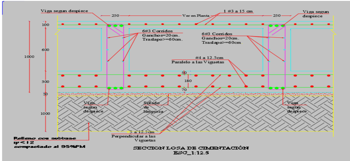
Ilustración 26. Disposición acero losa de cimentación
