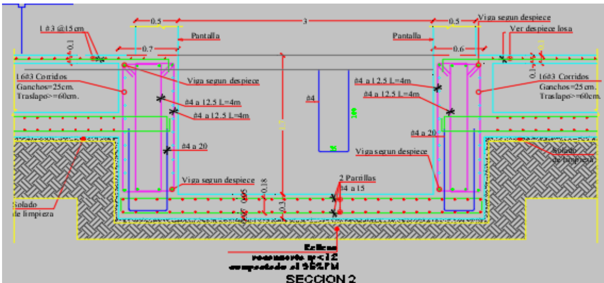
Ilustración 27. Disposición de acero losa foso ascensor
