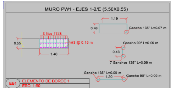
Ilustración 12. Disposición refuerzo pantalla PW1
