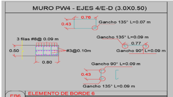
Ilustración 15. Disposición refuerzo pantalla PW4
