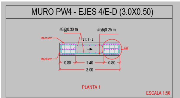
Ilustración 15. Disposición refuerzo pantalla PW4
