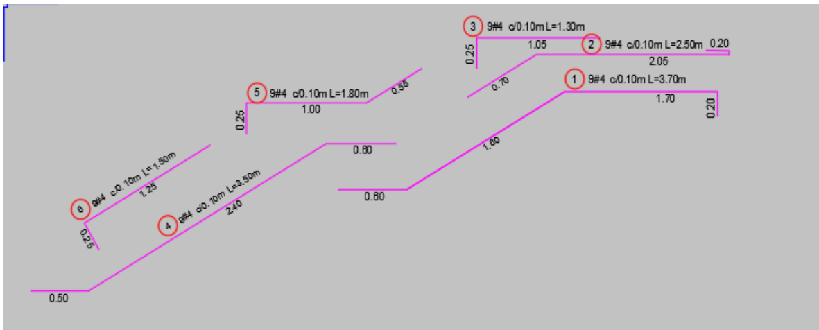
Ilustración 23 Disposición acero grada de emergencia.
