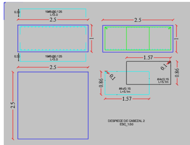
Ilustración 9. Disposición refuerzo Cabezal 2
