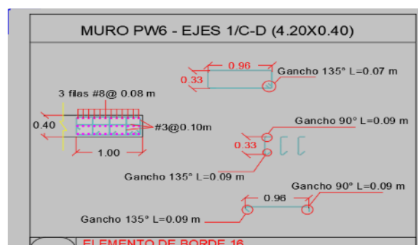
Ilustración 17. Disposición refuerzo pantalla PW6
