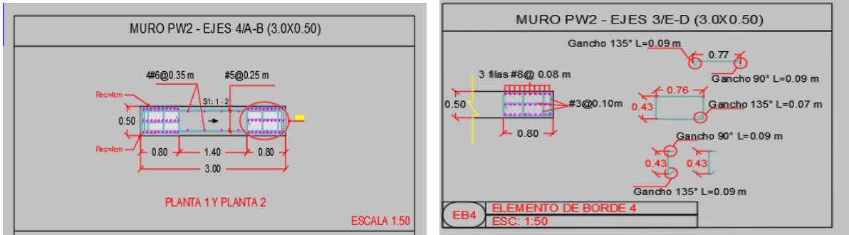
Ilustración 13. Disposición refuerzo pantalla PW2
