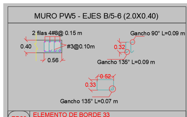
Ilustración 16. Disposición refuerzo pantalla PW5
