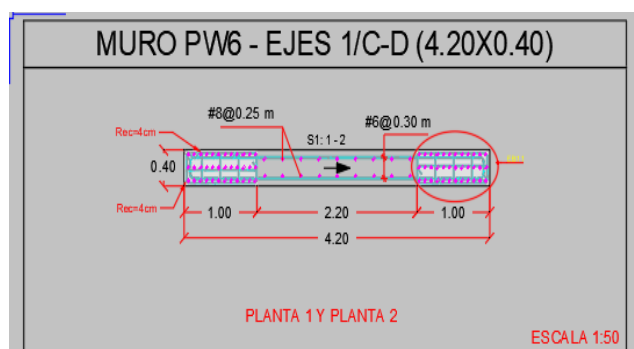
Ilustración 17. Disposición refuerzo pantalla PW6
