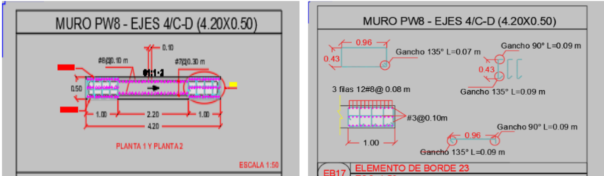
Ilustración 19. Disposición refuerzo pantalla PW8.
