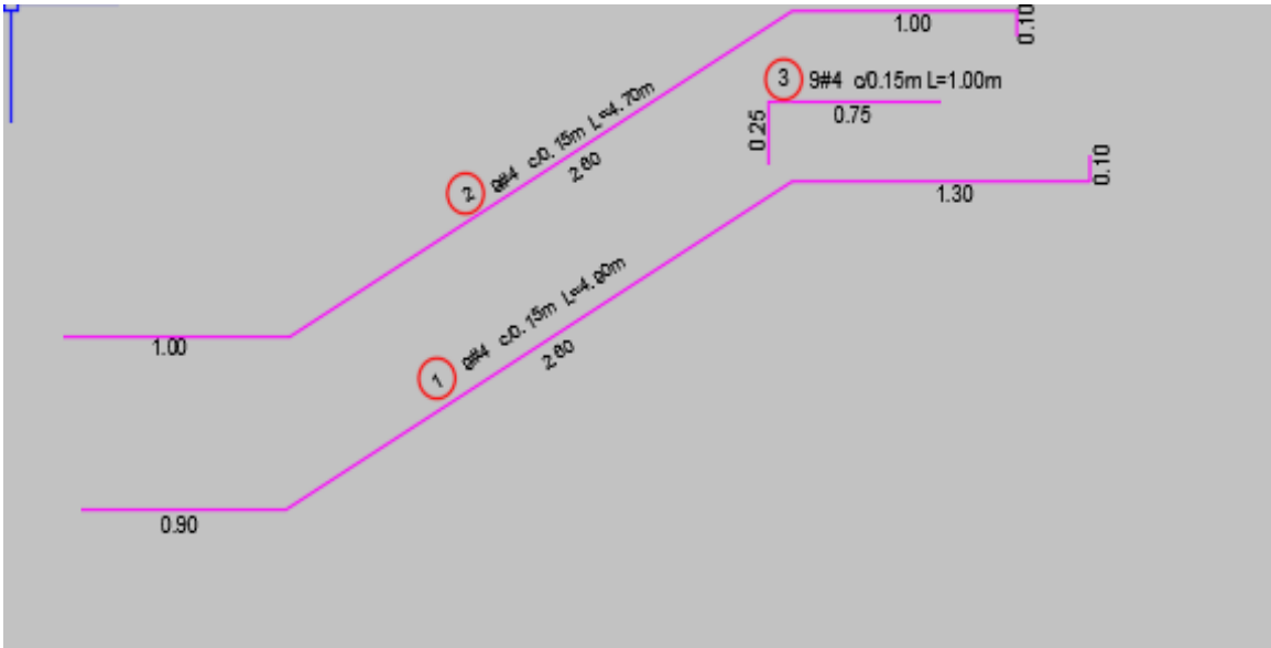
Ilustración 25 Disposición acero grada principal.
