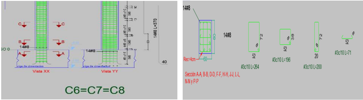
Ilustración 6. Disposición refuerzo columna C6,C7,Y C8
