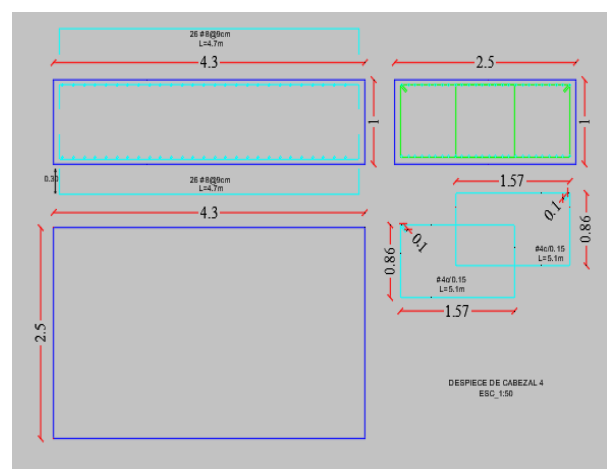
Ilustración 11. Disposición refuerzo Cabezal 4
