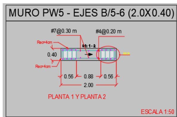
Ilustración 16. Disposición refuerzo pantalla PW5
