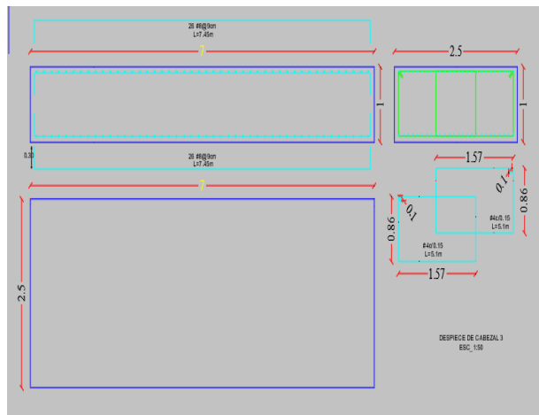
Ilustración 10. Disposición refuerzo Cabezal 3
