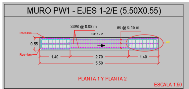
Ilustración 12. Disposición refuerzo pantalla PW1
