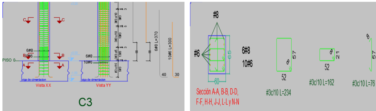
Ilustración 5. Disposición refuerzo columna C3.
