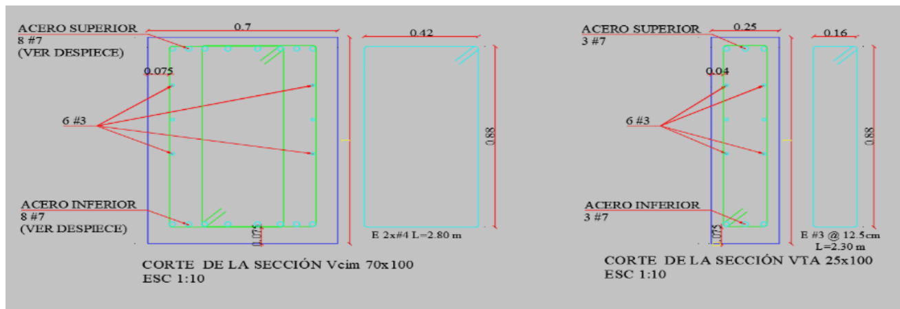
Ilustración 2. Disposición refuerzo vigas de cimentación y viguetas
