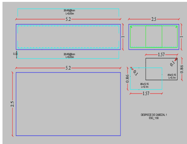
Ilustración 8. Disposición refuerzo Cabezal 1
