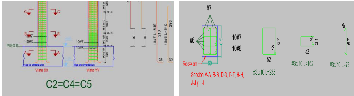
Ilustración 4. Disposición refuerzo columna C2, C4 y C5
