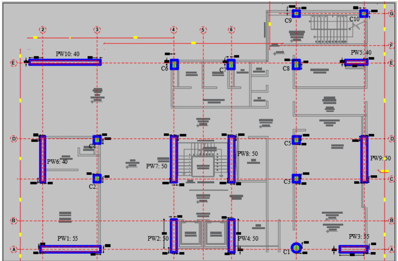
Ilustración 29. Localización ejes de pantallas y columnas
