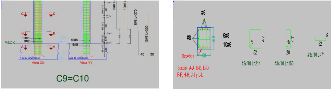
Ilustración 7. Disposición refuerzo columna C9 Y C10
