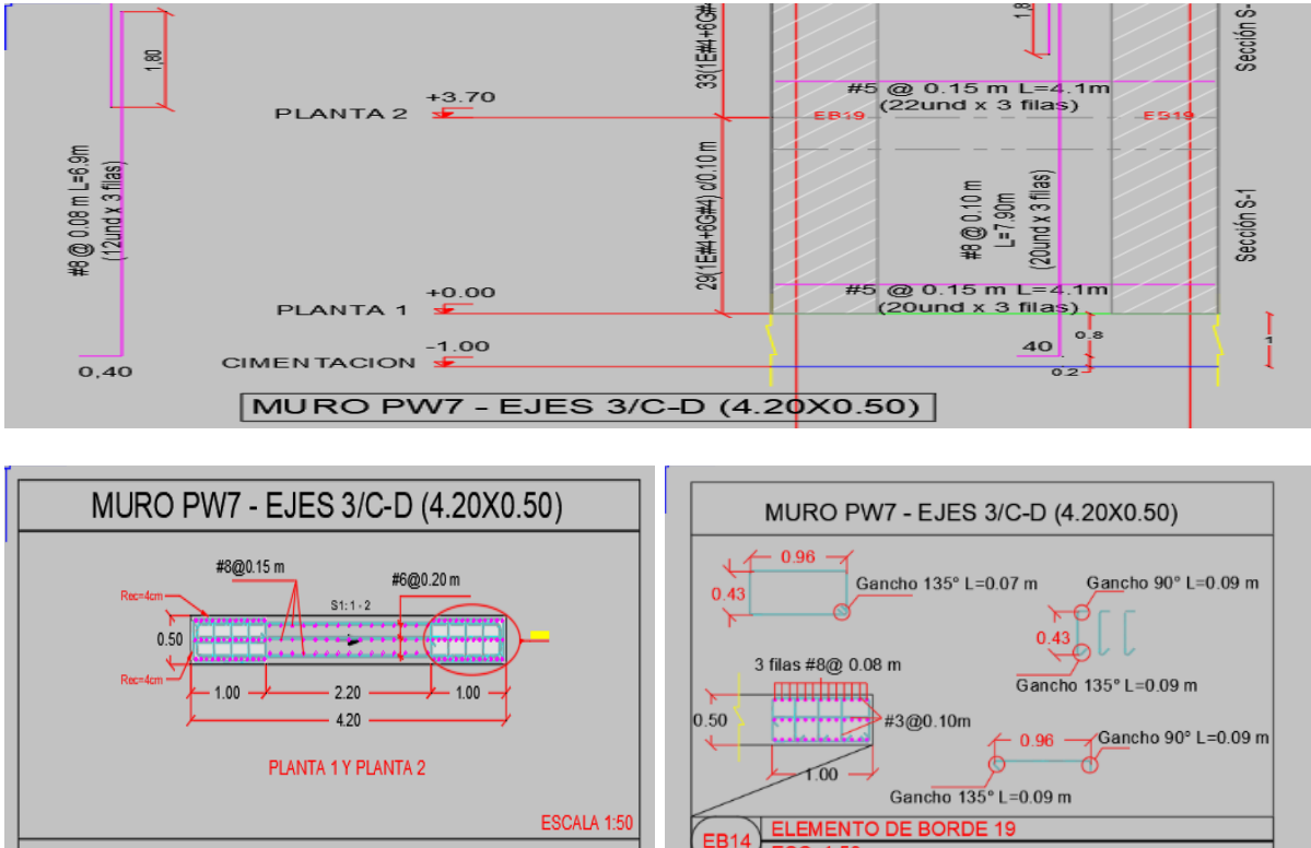
Ilustración 18. Disposición refuerzo pantalla PW7
