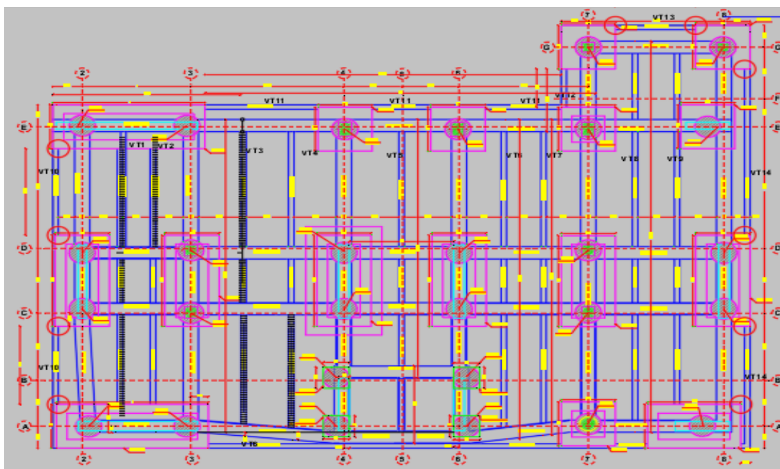
Ilustración 28. Localización ejes de cimentación, dados, vigas y viguetas
