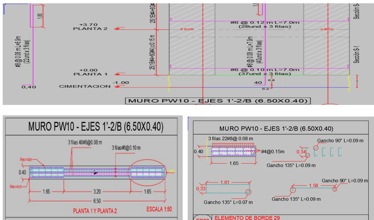
Ilustración 21. Disposición acero pantalla PW10.
