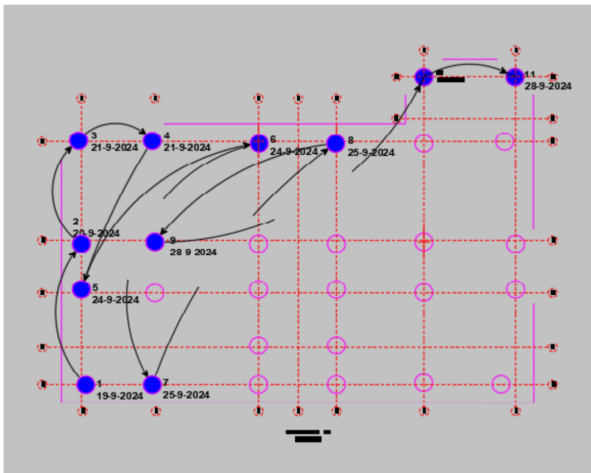
Ilustración 12. Secuencia de fundición de pilotes
