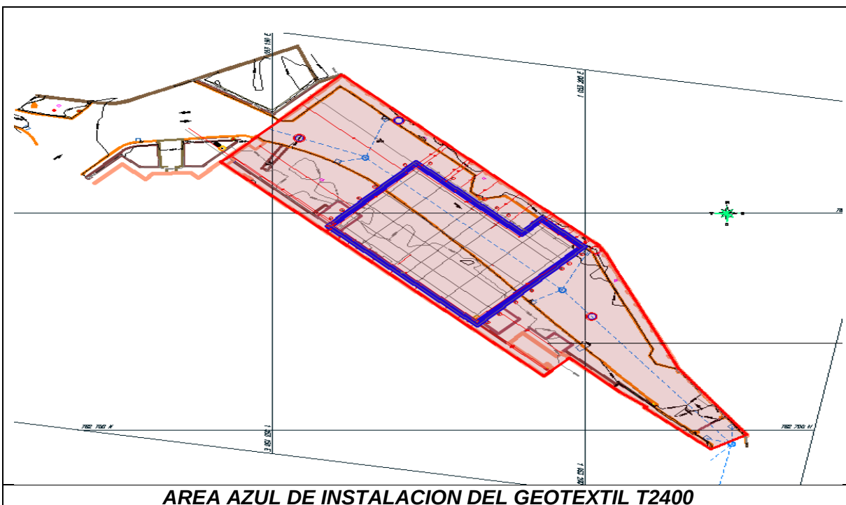
Ilustración 4. Área instalación geotextil T2400
