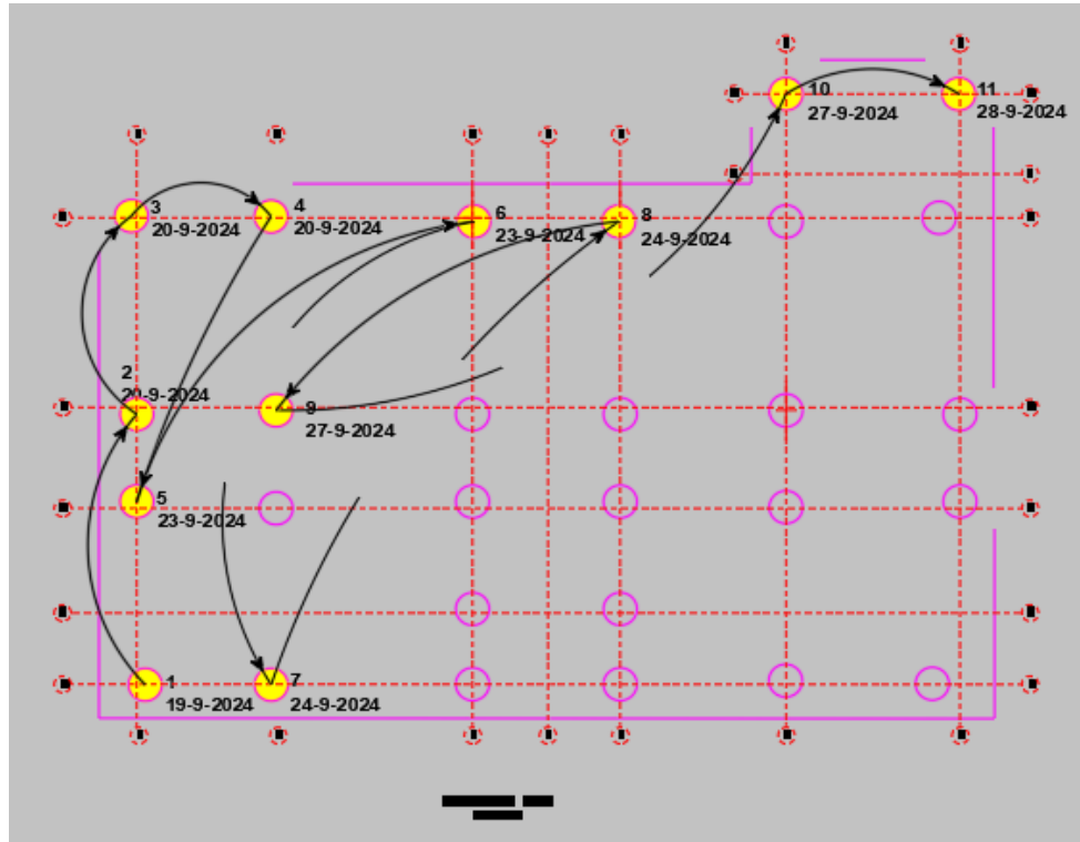
Ilustración 10. Secuencia excavación de pilotes
