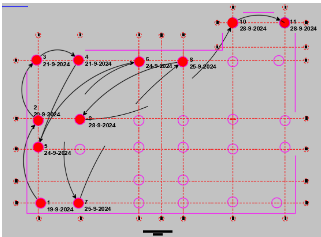
Ilustración 11. Secuencia instalación de acero pilotes
