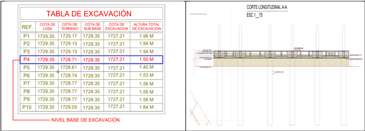
Ilustración 2. Niveles de excavación de cimentación del proyecto
