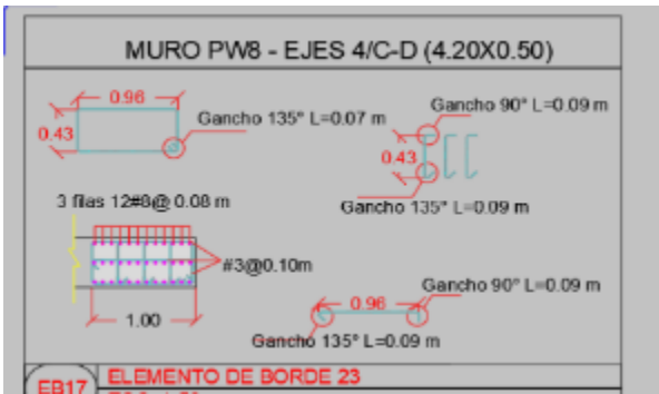
Ilustración 17. Disposición de refuerzo de pantalla PW8, piso 1
