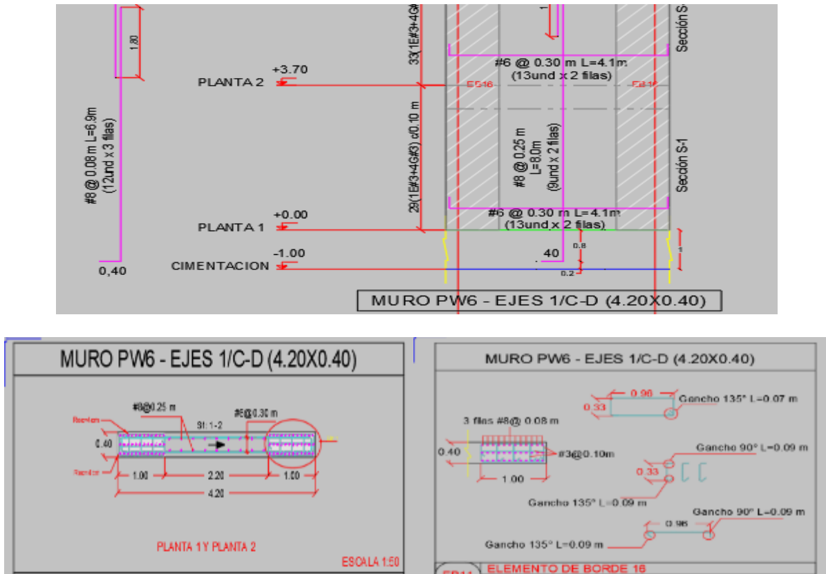
Ilustración 15. Disposición de refuerzo de pantalla PW6, piso 1
