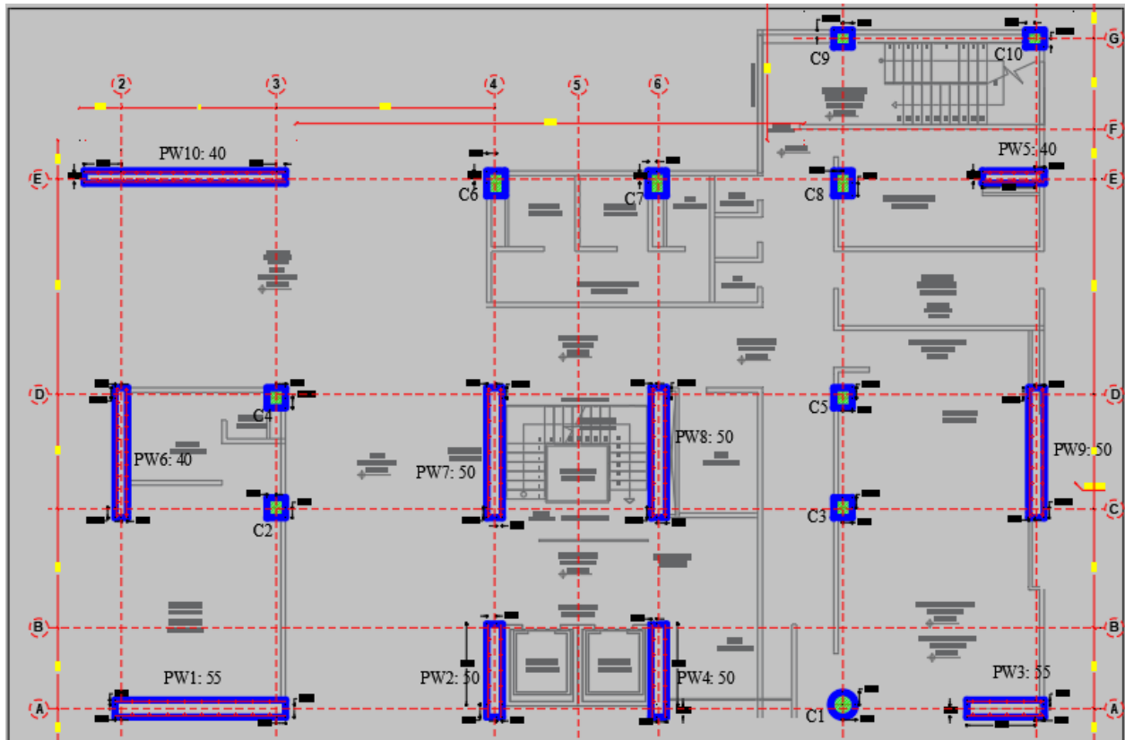
Ilustración 13. Localización ejes de pantallas y columnas
