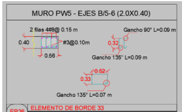
Ilustración 8. Disposición concreta PW5
