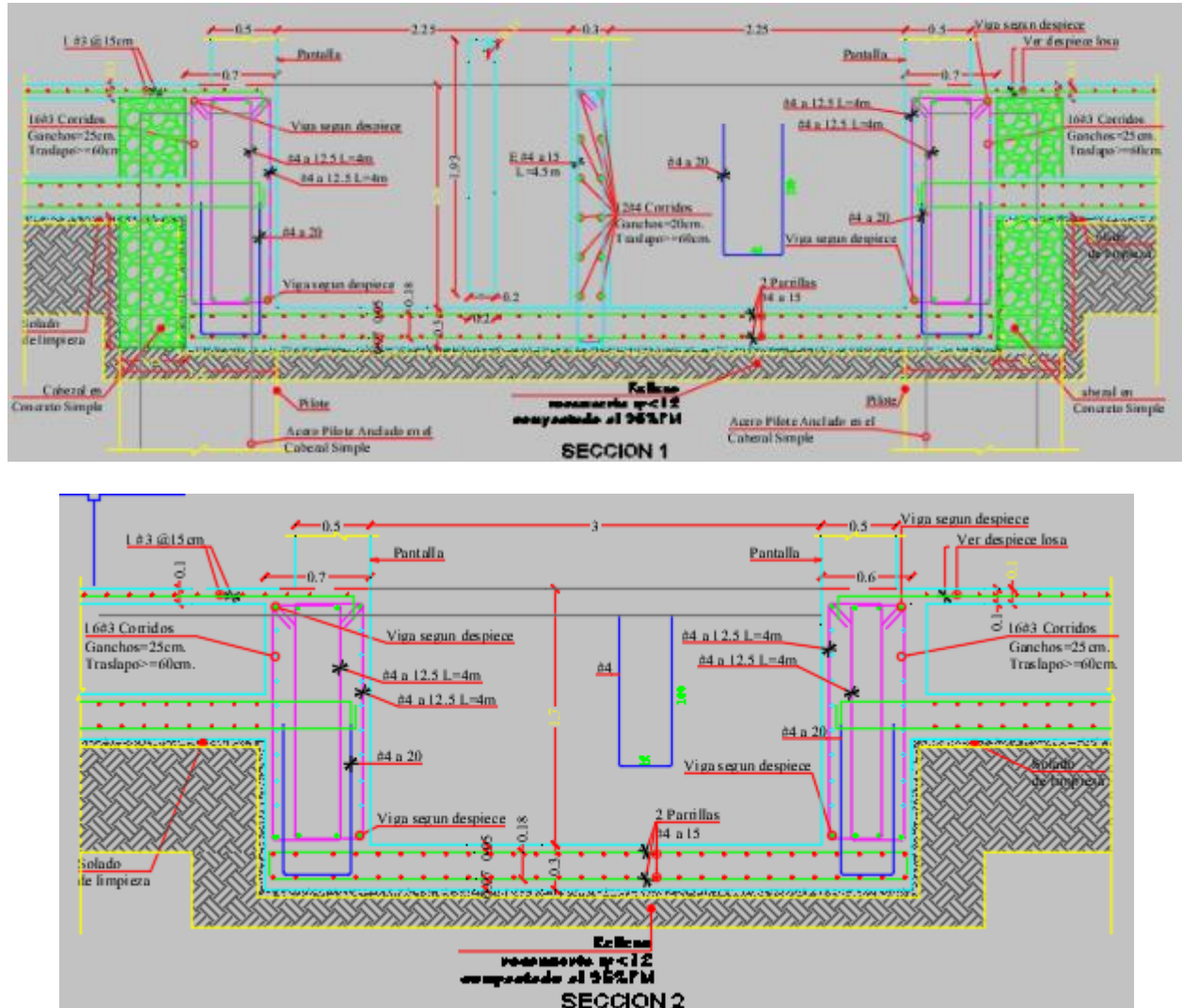
Ilustración 11. Disposición concretos foso ascensor
