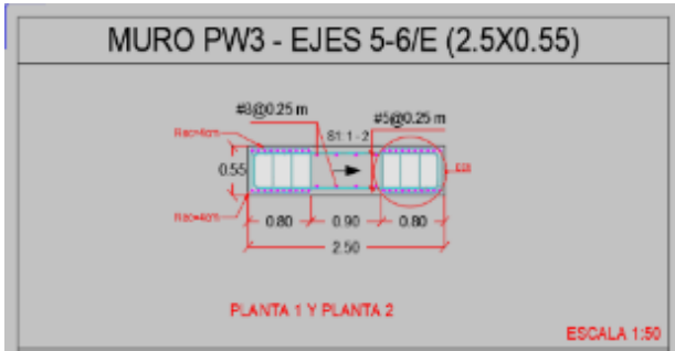
Ilustración 7. Disposición concreta PW3
