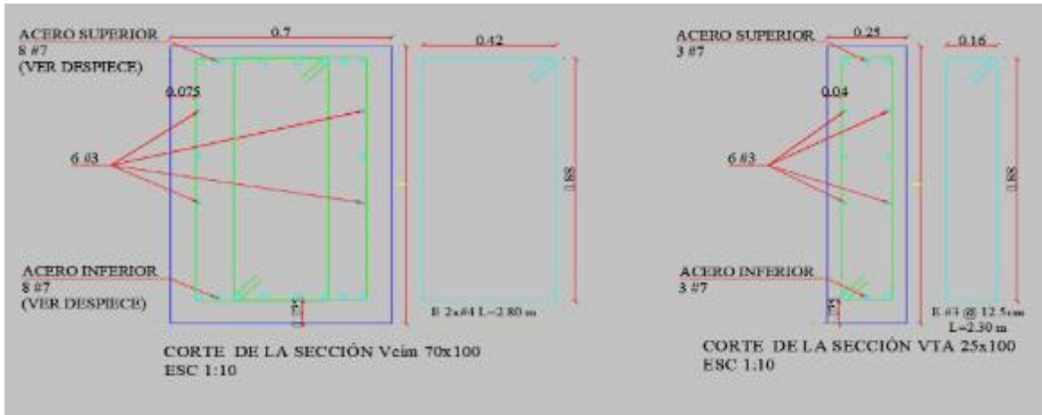
Ilustración 2. Disposición acero de refuerzo vigas y viguetas
