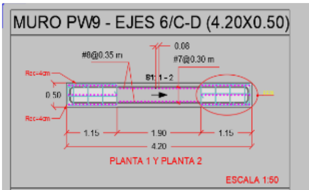
Ilustración 18. Disposición de refuerzo de pantalla PW9, piso 1
