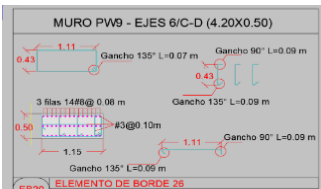
Ilustración 18. Disposición de refuerzo de pantalla PW9, piso 1
