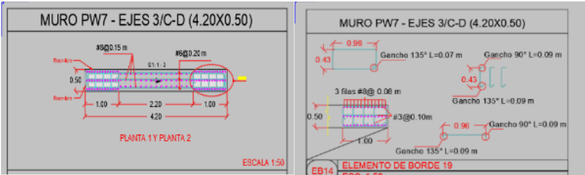
Ilustración 16. Disposición de refuerzo de pantalla PW7, piso 1
