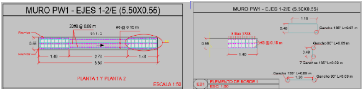
Ilustración 14. Disposición de refuerzo de pantalla PW1, piso 1
