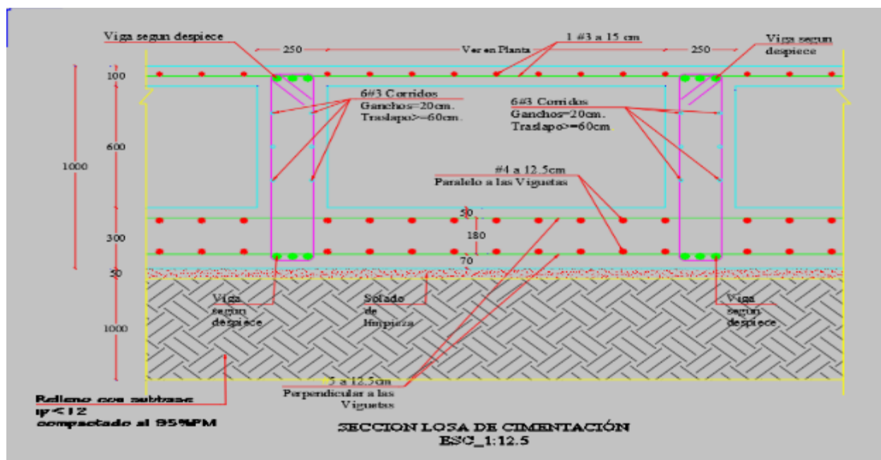
Ilustración 10. Disposicion acero de refuerzo losa de cimentación
