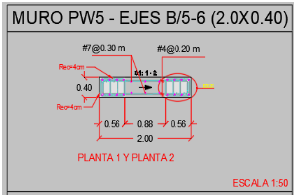
Ilustración 8. Disposición concreta PW5
