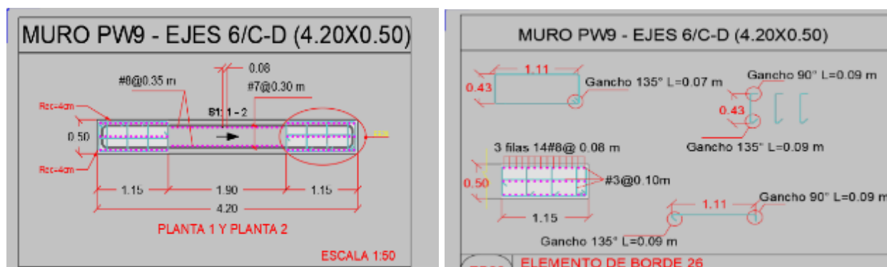
Ilustración 9. Disposición de concreto PW9
