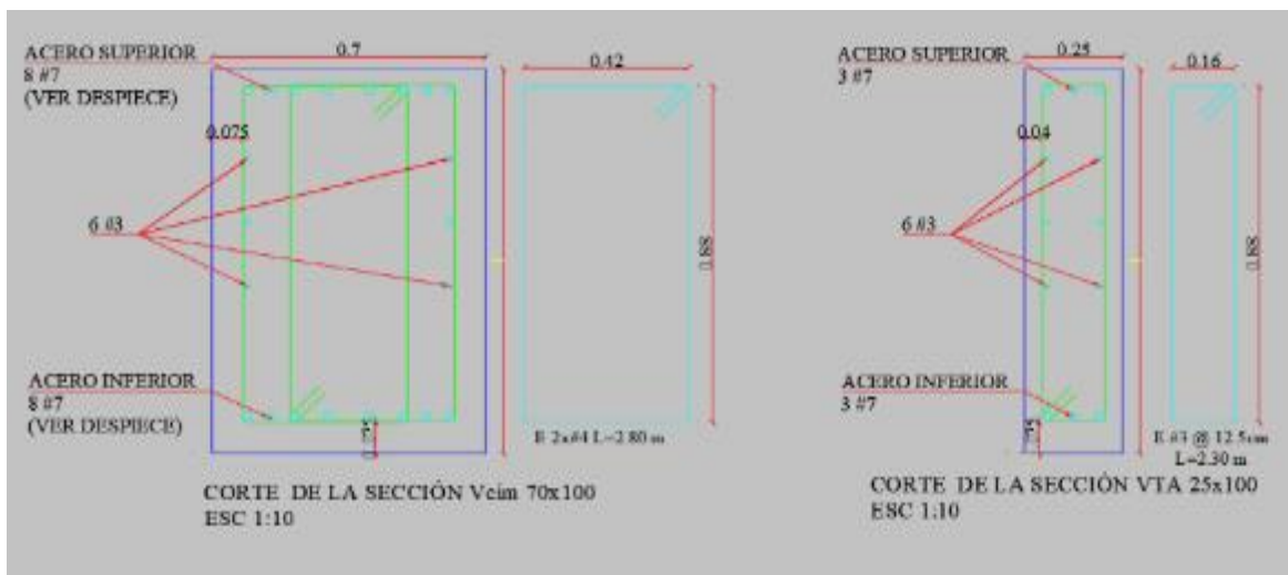
Ilustración 4. Disposición de concreto vigas y viguetas
