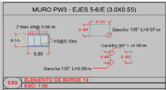
Ilustración 7. Disposición concreta PW3
