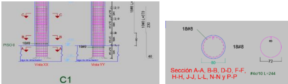
Ilustración 3. Disposición acero de refuerzo columna C1
