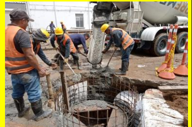
INSTALACION DE TUBERIA PLUVIAL 27" FUNDICION DE RECAMARAS
